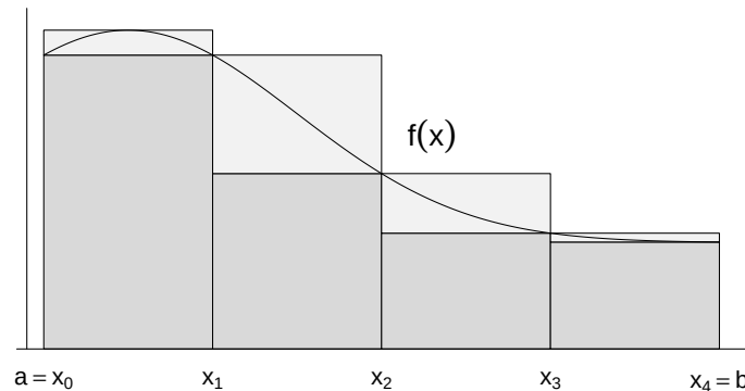
Abbildung 1.2. Riemannsche Summen
