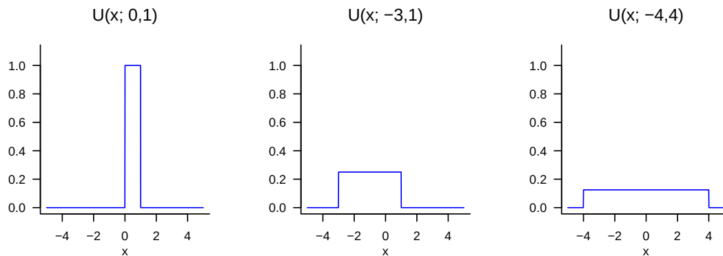
Abbildung 19.9. WDFen von gleichverteilten-Zufallsvariablen.
