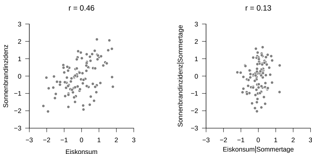
Abbildung 41.3. Evaluation der partiellen Korrelation im Beispielszenario.
