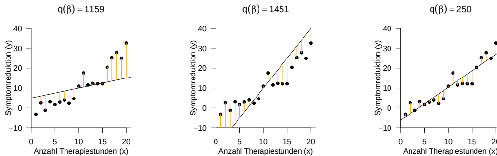
Abbildung 32.3. Vertikale Abweichungen und Quadratsummen bei unterschiedlichen Parameterwerten.
