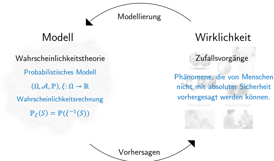
Abbildung 16.5. Wahrscheinlichkeitstheorie als Modell von Zufallsvorgängen. Ausgangspunkt der Wahrscheinlichkeitstheorie ist die Absicht, über einen Zufallsvorgang, also ein mit Unsicherheit behaftetes Phänomen der Wirklichkeit, logisch-quantitative Schlüsse zu ziehen. Die Repräsentation zentraler Aspekte des Zufallsvorgangs mithilfe wahrscheinlichkeitstheoretischer Begrifflichkeiten bezeichnet man als Modellierung. Das wahrscheinlichkeitstheoretische Modell selbst garantiert dann im Sinne der Wahrscheinlichkeitsrechnung die Korrektheit logisch-quantitativer Schlussfolgerungen, welche zur Vorhersage von Aspekten des Zufallsvorgangs genutzt werden können.
