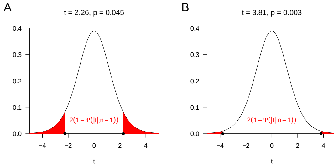
Abbildung 31.5. p-Werte für zwei mögliche Werte der Einstichproben-T-Test-Statistik bei n = 12 . Die Bereiche im Ergebnisraum der Einstichproben-T-Test-Statistik über denen roten Flächen eingezeichnet sind, markieren die Bereiche mit T \geq |t| gilt. Die summierten ihnen zugeordneten Wahrscheinlichkeiten, also die entsprechenden roten Flächen unter der WDF der t -Verteilungen entsprechen dem p-Wert
