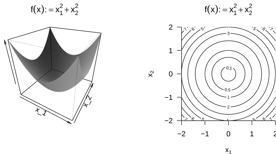
Abbildung 6.5. Visualisierungen einer bivariaten Funktion.
