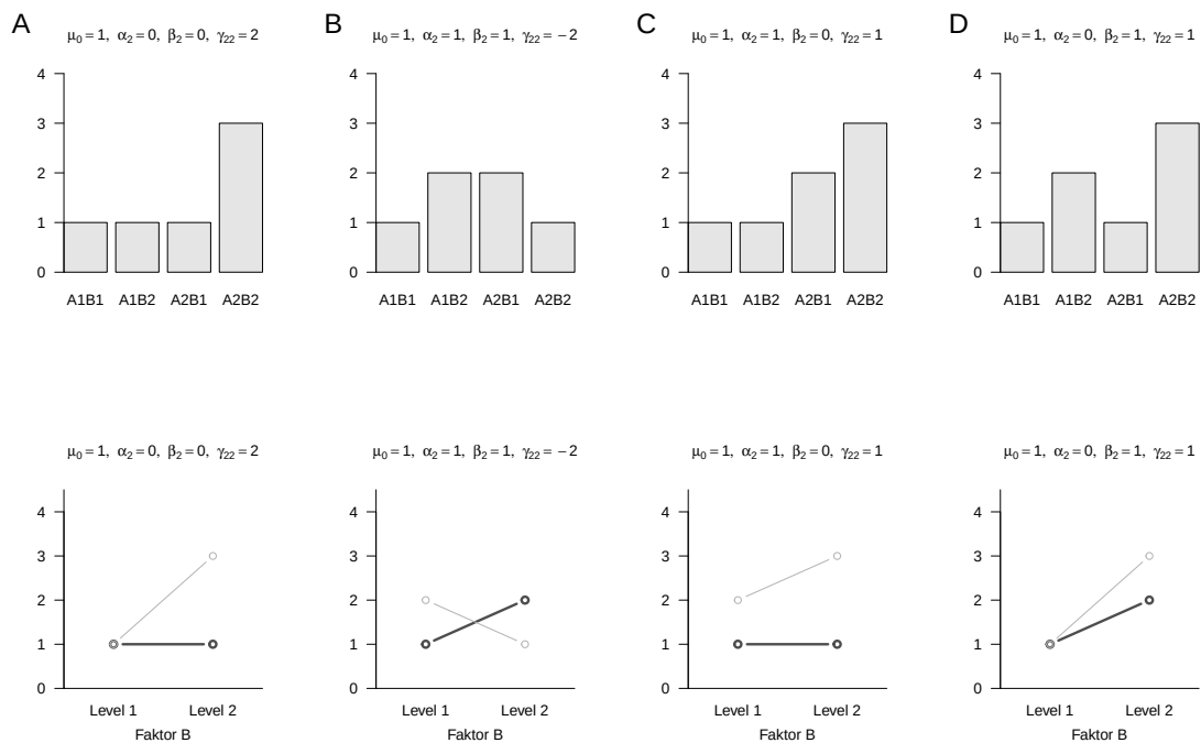
Abbildung 40.5. Gruppenerwartungswerte der Beispielparameterszenarien in Balken- und Liniendiagrammform im Modell der ZVA mit Interaktion.
