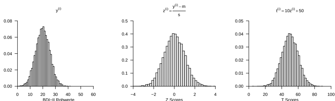
Abbildung 47.2. Simulierte Stichproben-BDI-II Rohwerte, Z Scores und T Scores
