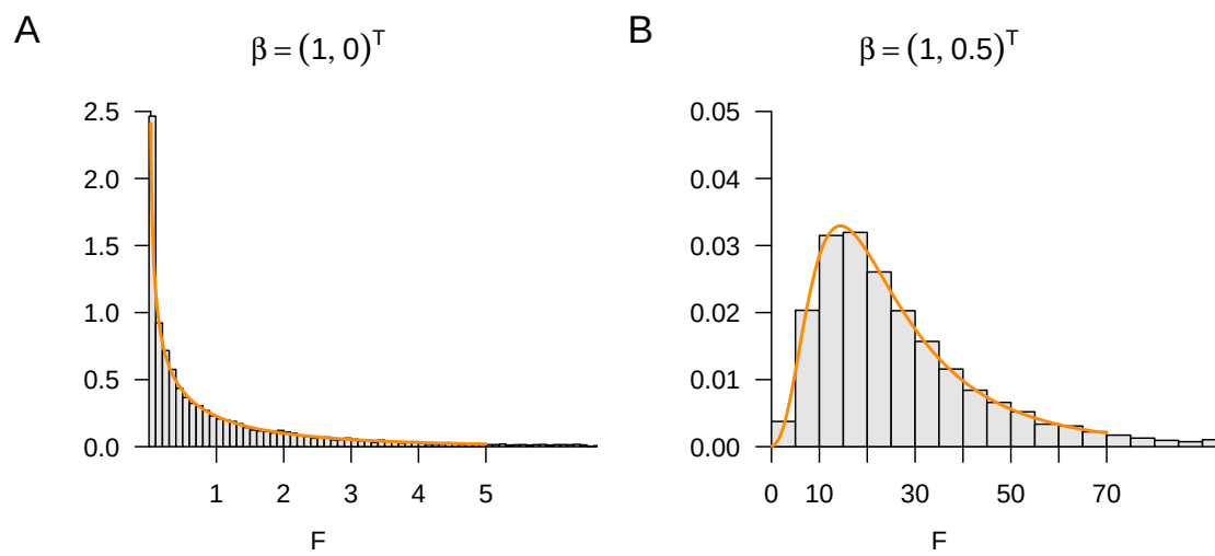
Abbildung 37.2. Exemplarische F-Statistik Verteilungen unter reduziertem und vollständigem wahren, aber unbekanntem, datenerzeugenden Modell bei einfacher linearer Regression.
