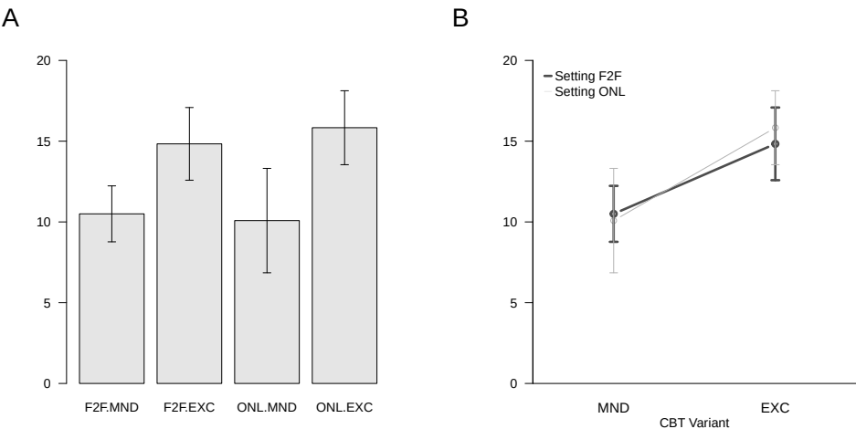
Abbildung 40.3. Visualisierung des Beispieldatensatzes als Balken- und Liniendiagramm.
