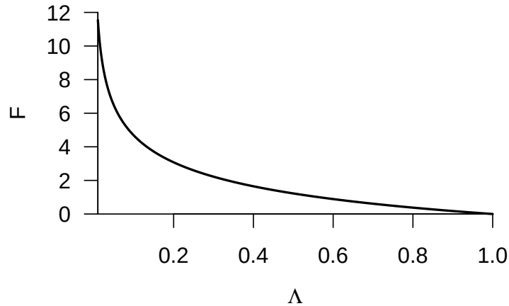
Abbildung 37.1. Zusammenhang von F- und Likelihood-Quotienten-Statistik.
