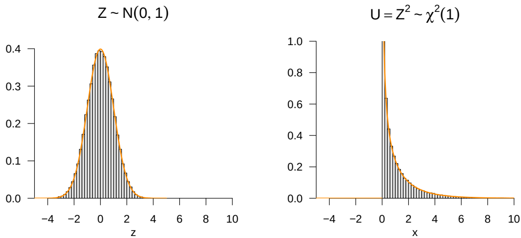
Abbildung 27.13. \chi^2 -Transformation normalverteilter Zufallsvariablen.
