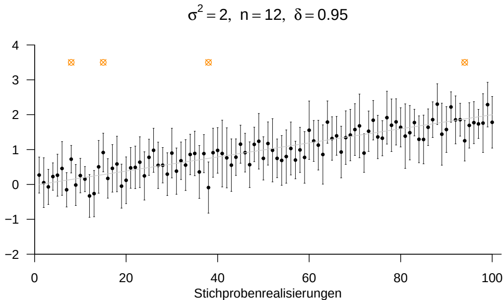
Abbildung 30.4. Simulation der Überdeckungswahrscheinlichkeit des Konfidenzintervalls für den Erwartungswertparameter des Normalverteilungsmodells bei variablem, wahren, aber unbekannten, Erwartungswertparameter \mu für \sigma^2 := 2, n := 12 und einer gewünschten Überdeckungswahrscheinlichkeit von \delta := 0.95 . Die Abbildung zeigt für jede Stichprobenrealisierung das Konfidenzintervall und den entsprechenden Erwartungswertparameterschätzer. In der vorliegenden Simulation überdecken die Konfidenzintervalle den durch eine graue Linie eingezeichneten variablen wahren, aber unbekannten, Erwartungswertparameter \mu in 95 von 100 Fällen. Die Stichprobenrealisierungen, für die dies nicht der Fall ist, sind mit einem orangen Kreis markiert
