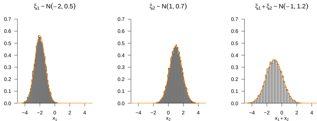
Abbildung 27.9. Summation normalverteilter Zufallsvariablen.
