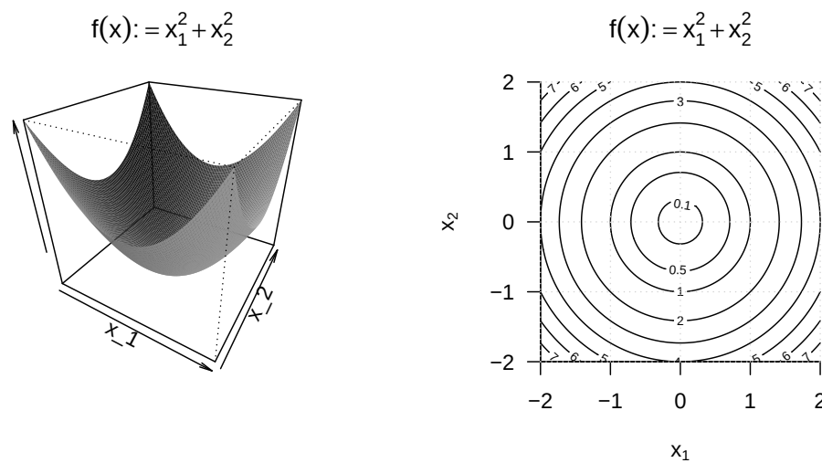
Abbildung 6.5. Visualisierungen einer bivariaten Funktion. Die linke Darstellung visualisiert die Funktionswerte als Fläche über der zweidimensionalen Definitionsmenge der Funktion. Auch wenn diese Darstellung einen gewissen dreidimensionalen Charakter hat, handelt es sich um eine bivariate Funktion mit entsprechend zweidimensionaler Definitionsmenge. Die rechte Abbildung visualisiert Linien mit gleichen Funktionswerten in der zweidimensionalen Definitionsmenge der Funktion.
