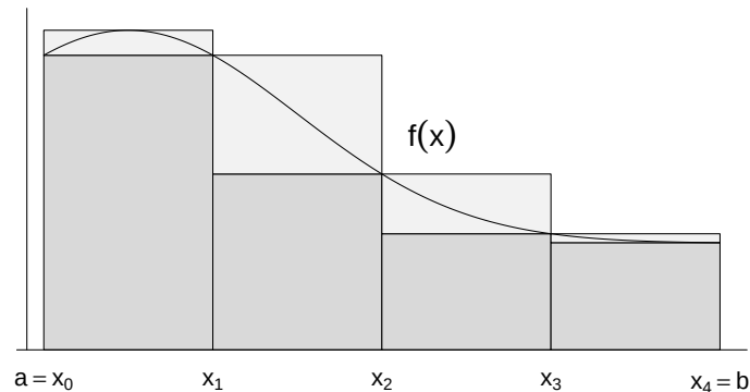
Abbildung 7.2. Riemannsche Summen
