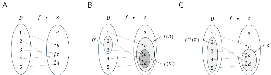
Abbildung 4.2. (A) Visualisierung der Funktion Gleichung 4.5. (B) Wertebereich und eine Bildmenge von f . (C) Urbildmenge einer Menge Z' unter f
