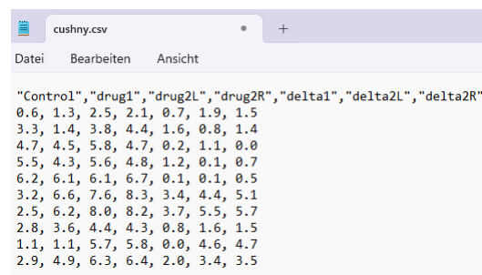
Textuelles Datenformat
