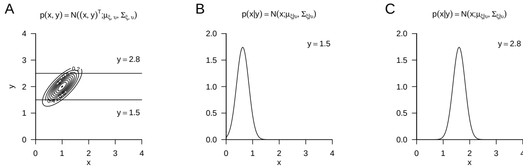
Abbildung 29.7. Bedingte Normalverteilungen
