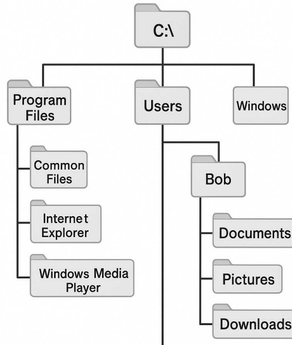
Abbildung 17.3. Windows Verzeichnisstruktur
