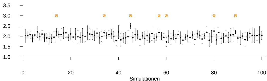
Abbildung 38.3. Konfidenzintervalle für Betaparameterkomponenten bei einfacher linearer Regression.
