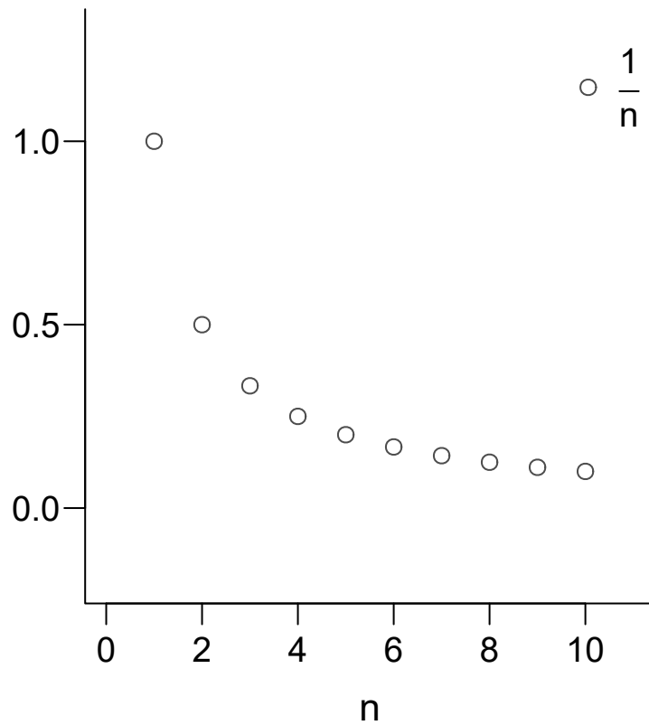
Harmonische Folge
