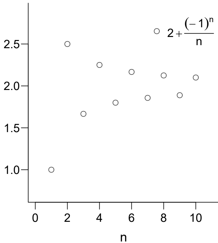
Sprungfolge
