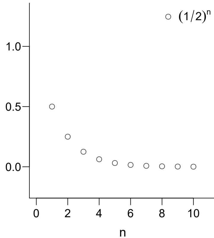
Geometrische Folge
