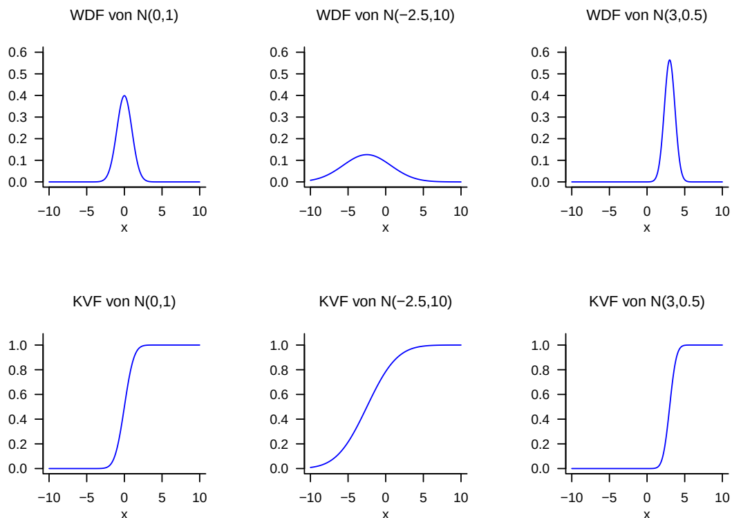
Abbildung 21.12. WDFen und KVFe von normalverteilten Zufallsvariablen.
