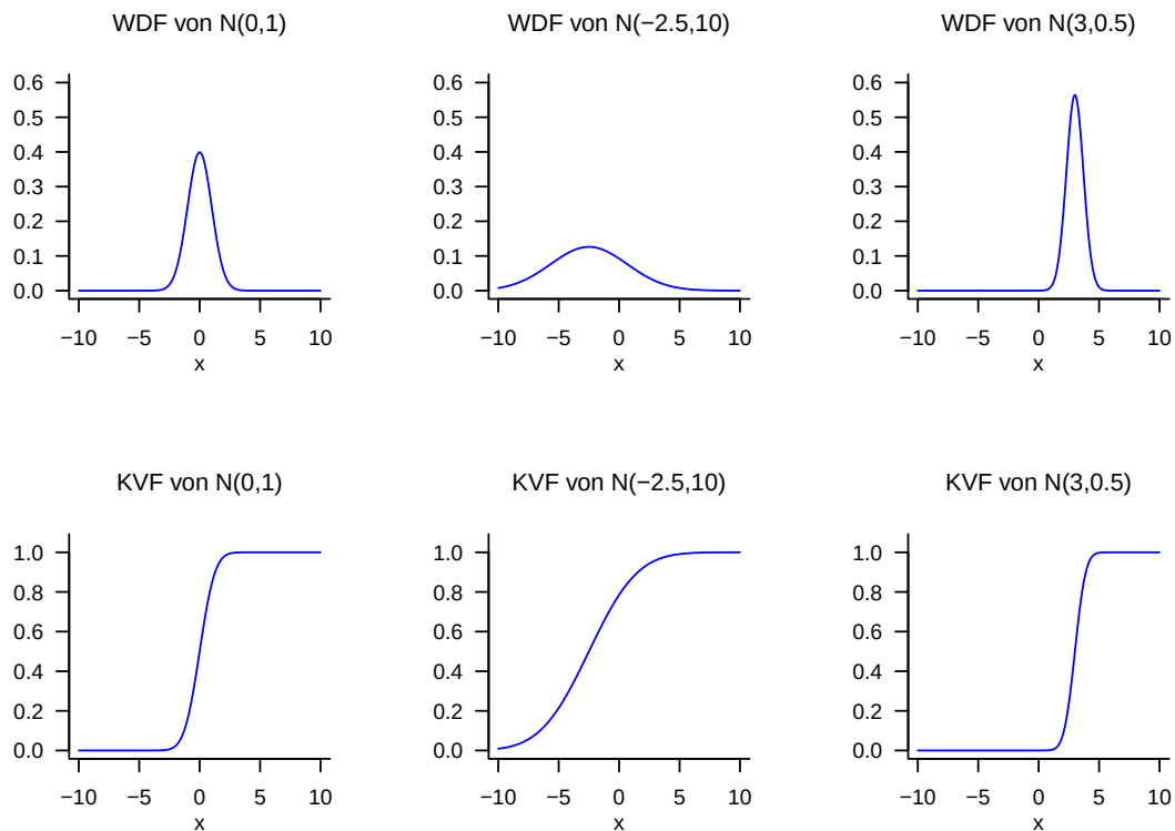
Abbildung 19.12. WDFen und KVFe von normalverteilten Zufallsvariablen.
