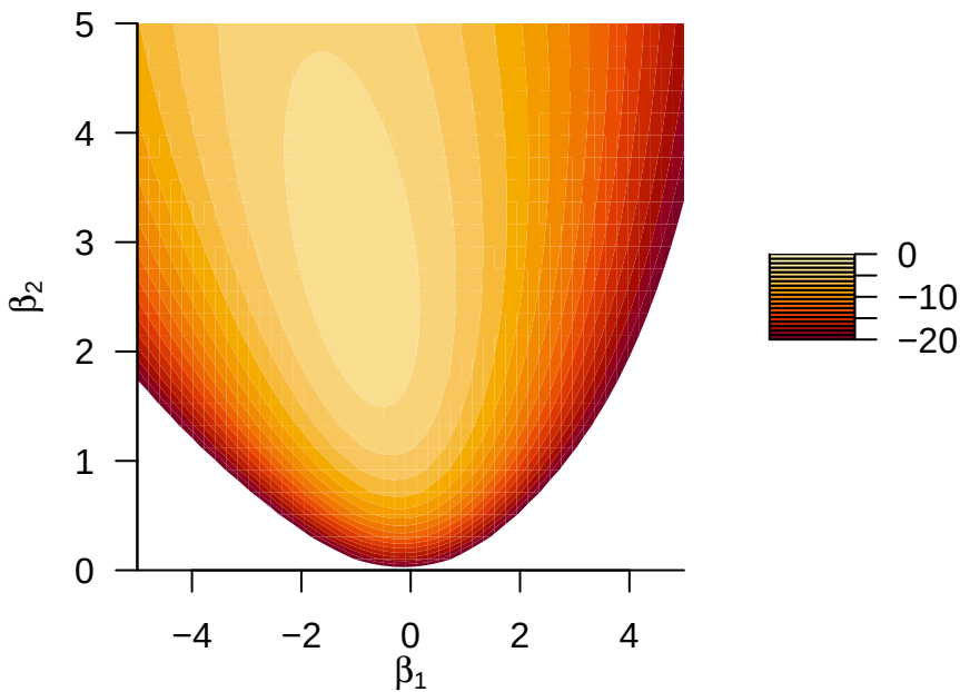
Log-Likelihood-Funktion
