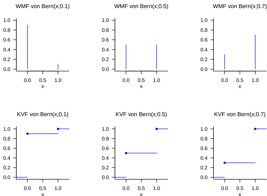
Abbildung 13.10. WMFe und KVFe von Bernoulli-Zufallsvariablen.
