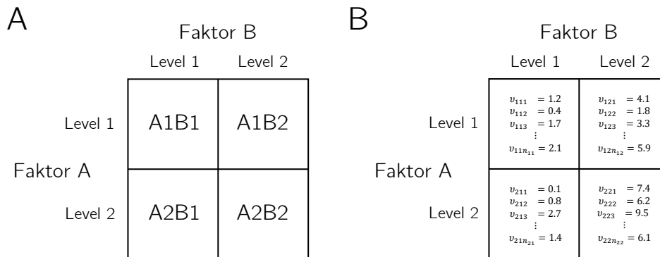
Abbildung 34.1. Konzeptuelles Design und Datennotation einer 2 \times 2 ZVA.
