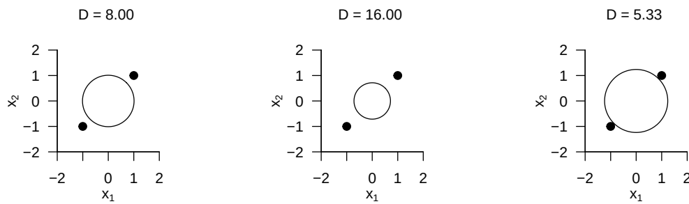
Abbildung 37.1. Mahalanobis-Distanzen als Funktion von Komponentenvarianzen
