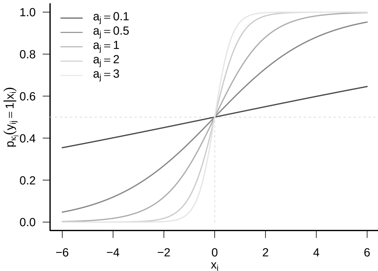
Effekt des Itemdiskriminationsparameters bei b_j = 0 , c_j = 0
