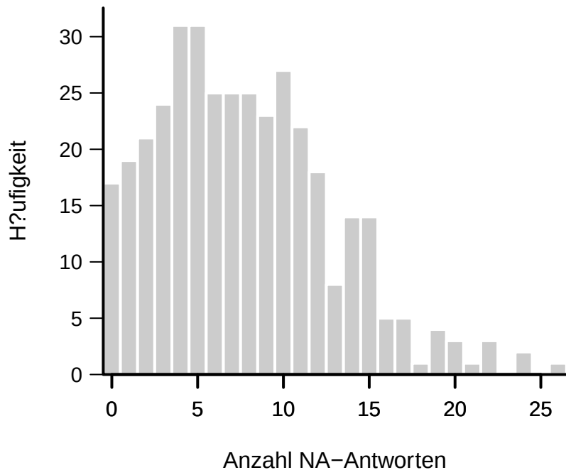
Personen (n = 369, NA-Mittel = 7.8)
