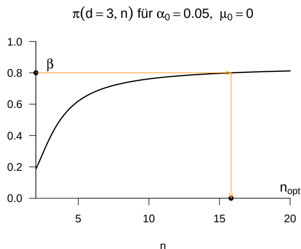
Abbildung 33.8. Praktische Durchführung einer Powerfunktionsbasierter Stichprobenumfangoptimierung. Bei gewählten Signifikanzlevel \alpha_0 und fest angenommenen Nichtzentralitätsparameter d^* evaluiert man den Stichprobenumfang für den die Testpowerfunktion einen Wert von \beta oder größer hat.
