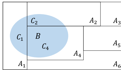
Abbildung 20.3. Venn-Diagramm zum Beweis von Theorem 20.4.
