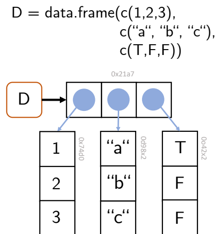
Abbildung 16.3. Dataframerepräsentation. Ein R Dataframe ist einer R Liste deren Elemente R Vektoren gleicher Länge sind.
