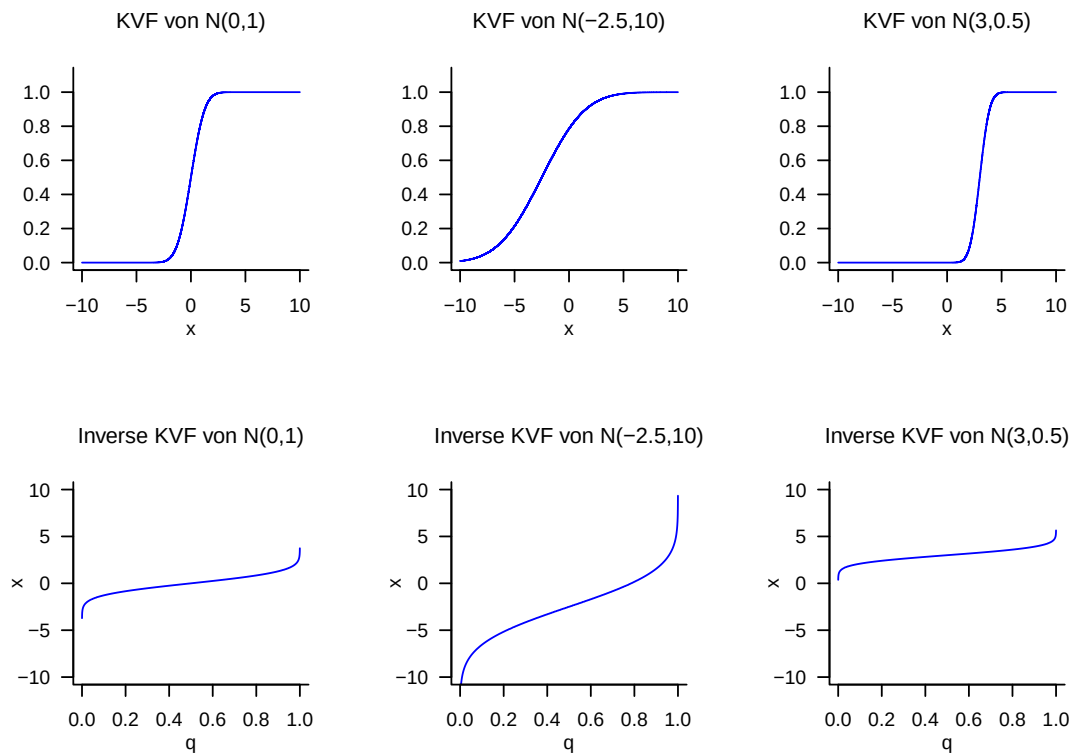
Abbildung 21.13. KVFe und inverse KVFe von normalverteilten Zufallsvariablen.
