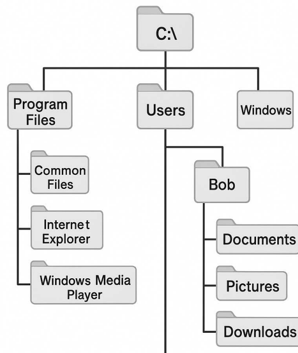
Abbildung 17.3. Windows Verzeichnisstruktur
