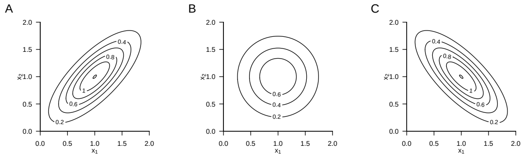
Abbildung 21.3. Wahrscheinlichkeitsdichtefunktionen bivariater Normalverteilungen.
