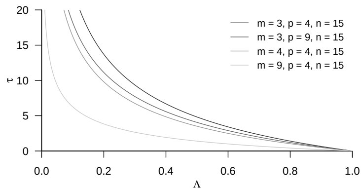
Abbildung 39.4. Beziehung der Wilks'- \Lambda -Statistik und der von Rao (1951) betrachteten \tau Statistik in exemplarischen Anwendungsszenarien.
