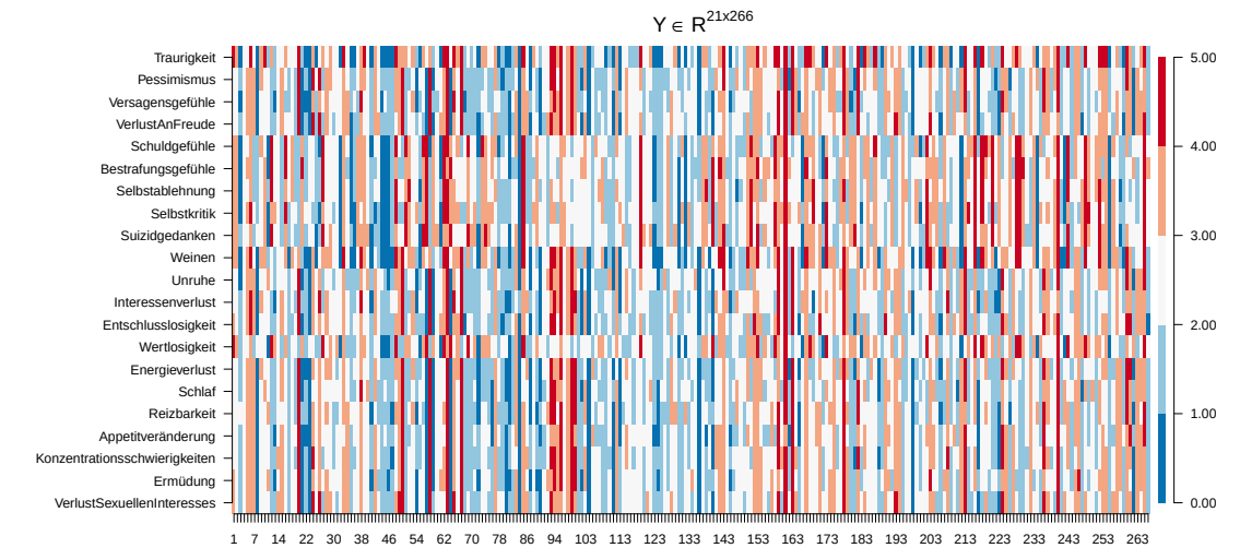
Abbildung 43.1. Simulierter BDI-II Datensatz nach Keller et al. (2008).
