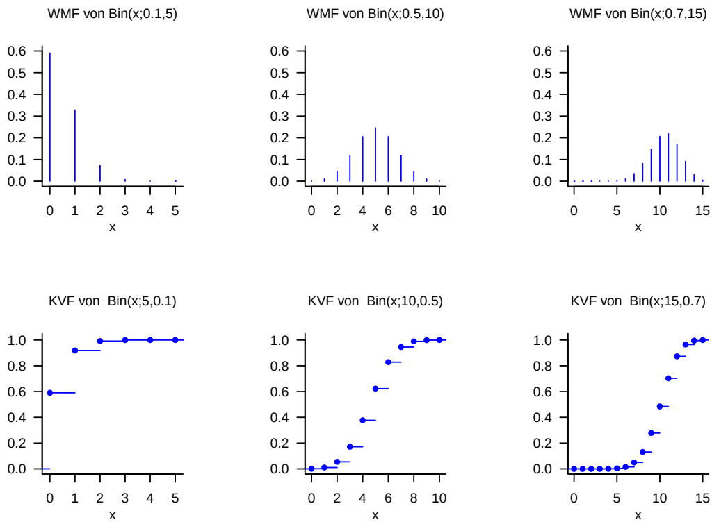
Abbildung 13.11. WMFen und KVFe von Binomial-Zufallsvariablen.
