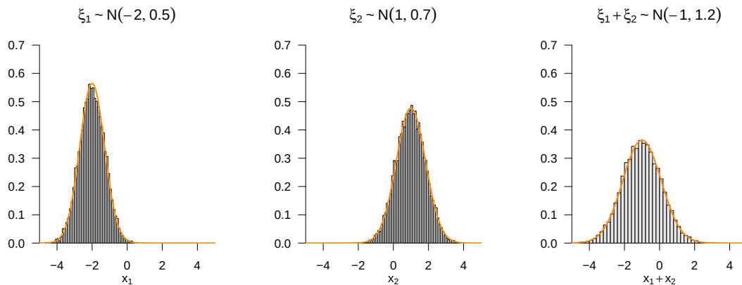
Abbildung 21.9. Summation normalverteilter Zufallsvariablen.
