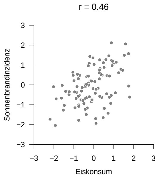
Abbildung 35.1. Beispielszenario zur Evaluation bedingter und partieller Korrelationen.
