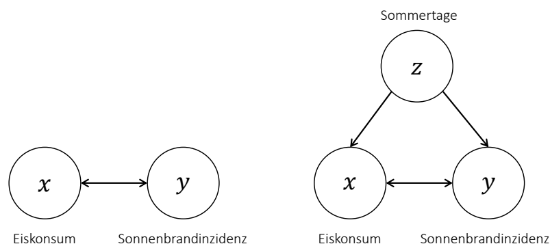
Abbildung 35.2. Zufallsvariablen im Beispielszenario.
