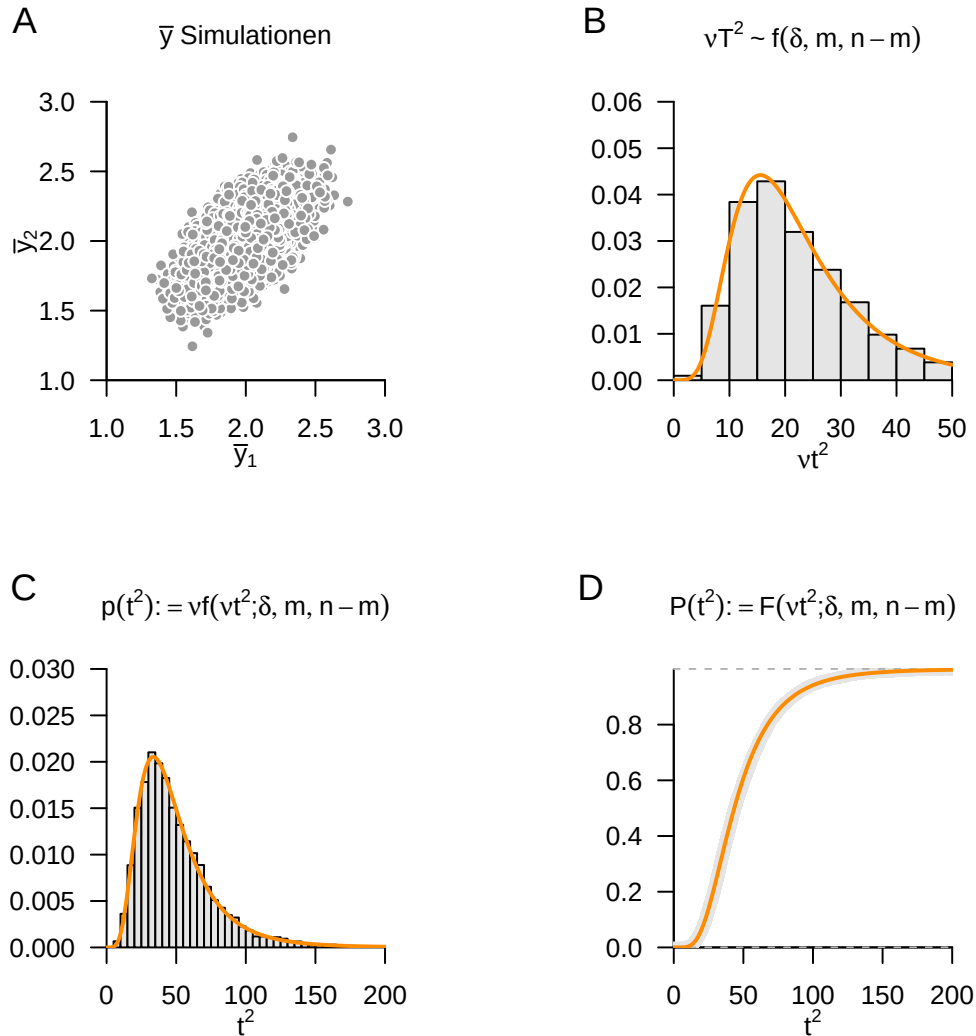
Abbildung 38.4. Verteilung der Einstichproben- T^2 -Teststatistik. A Stichprobenmittel von 10.000 Realisierungen eines Einstichproben- T^2 -Test-Modells mit m := 2 und n := 15 und wahren, aber unbekannten, Parametern
