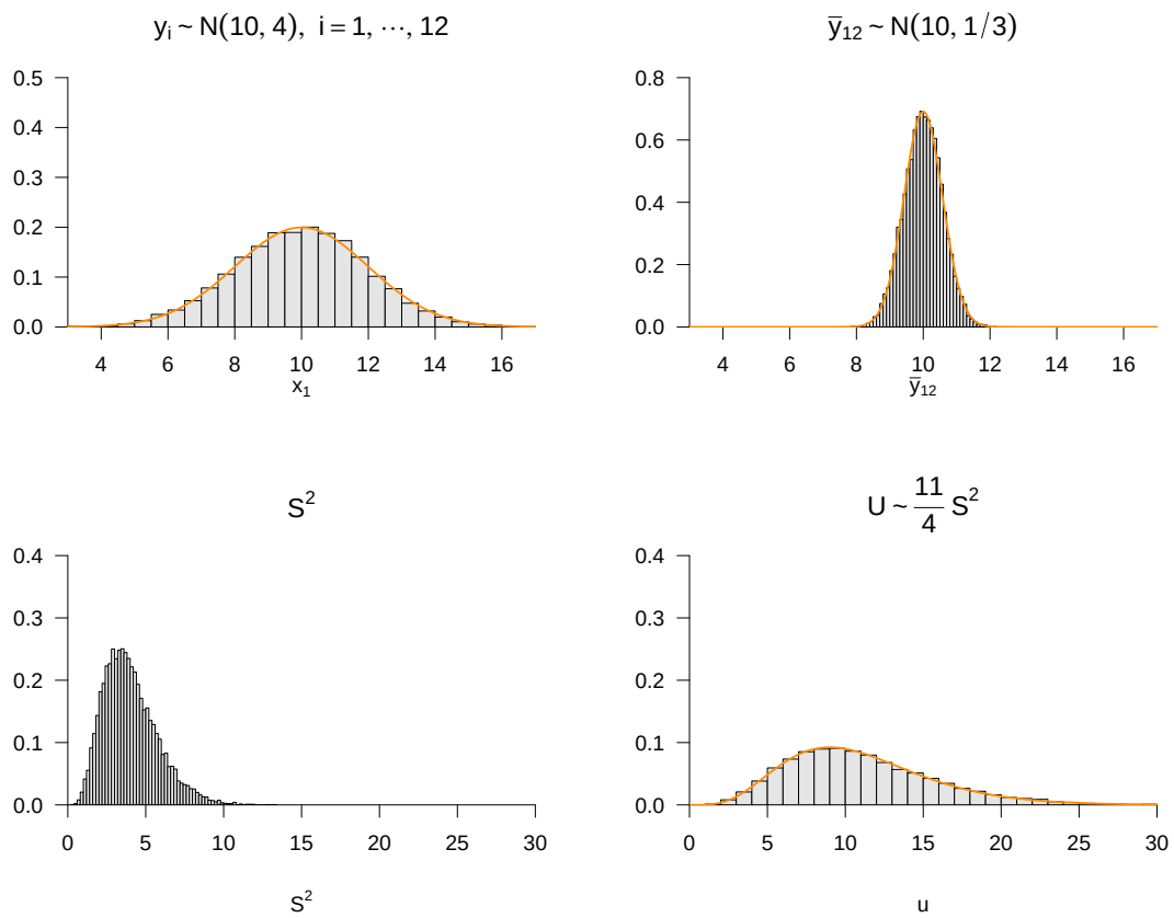
Abbildung 24.5. Simulation der Verteilung der U -Konfidenzintervallstatistik und der ihr zugrundeliegenden Verteilungen der Stichprobenvariable, des Stichprobenmittels und der Stichprobenvarianz.
