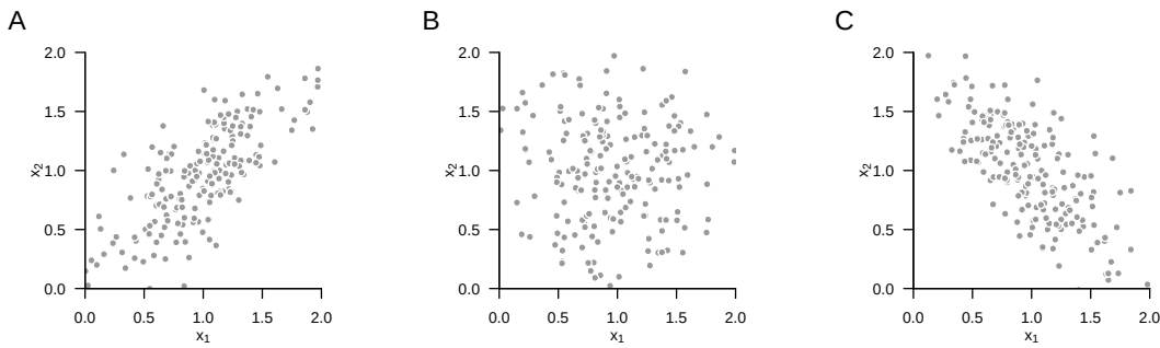
Abbildung 21.4. Realisierungen bivariat normalverteilter Zufallsvektoren.
