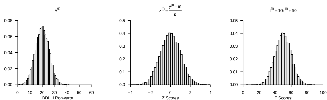
Abbildung 41.2. Simulierte Stichproben-BDI-II Rohwerte, Z Scores und T Scores
