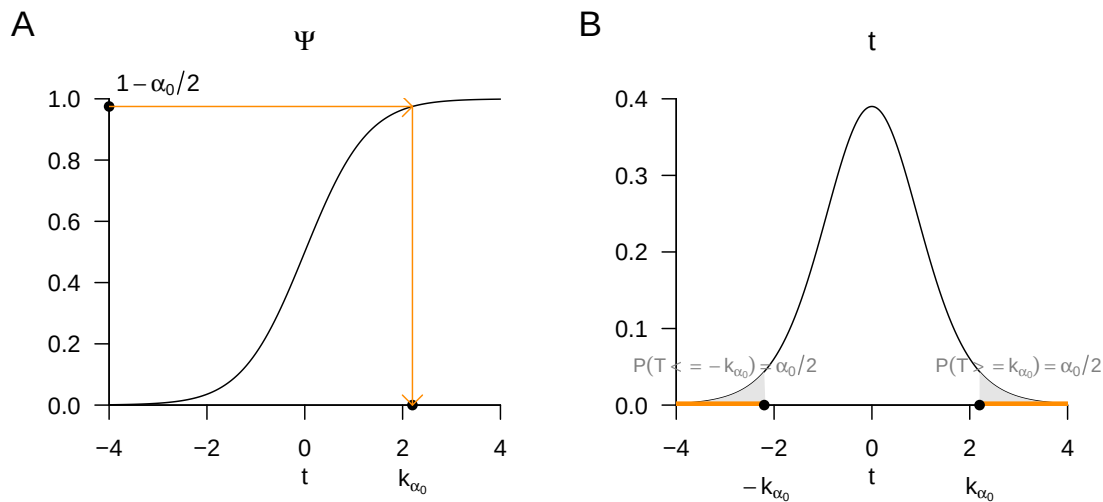
Abbildung 25.4. Bestimmung des kritischen Werts k_{\alpha_0} für den zweiseitigen Einstichproben-T-Tests mit einfacher Nullhypothese für n = 12 und \alpha_0 := 0.05 zu Kontrolle des Testumfangs (A) Für ein gewähltes \alpha_0 ist der kritische Wert des betrachteten Tests nach Theorem 25.3 durch den Wert der inversen KVF der t -Verteilung mit Freiheitsgradparameter n - 1 an der Stelle 1 - \frac{\alpha_0}{2} gegeben. Die Abbildung zeigt die Bestimmung dieses Werts zu k_{0.05} = 2.2 anhand der KVF der t -Verteilung mit Freiheitsgradparameter n - 1 . (B) Die Abbildung zeigt den aus der Wahl von k_{\alpha_0} resultierenden Ablehnungsbereich des betrachteten Tests als grau hinterlegte Flächen unter der WDF der t -Verteilung mit Freiheitsgradparameter n - 1 . Die symmetrische Verteilung der Teilmengen des Ablehnungsbereichs in den Ausläufern der WDF ergibt sich dabei aus der Definition des Tests als Funktion des Betrages der Einstichproben-T-Test-Statistik, also insbesondere des zweiseitigen Charakters des hier betrachteten Tests.
