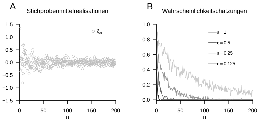
Abbildung 19.1. Simulation des schwachen Gesetz der Großen Zahlen.
