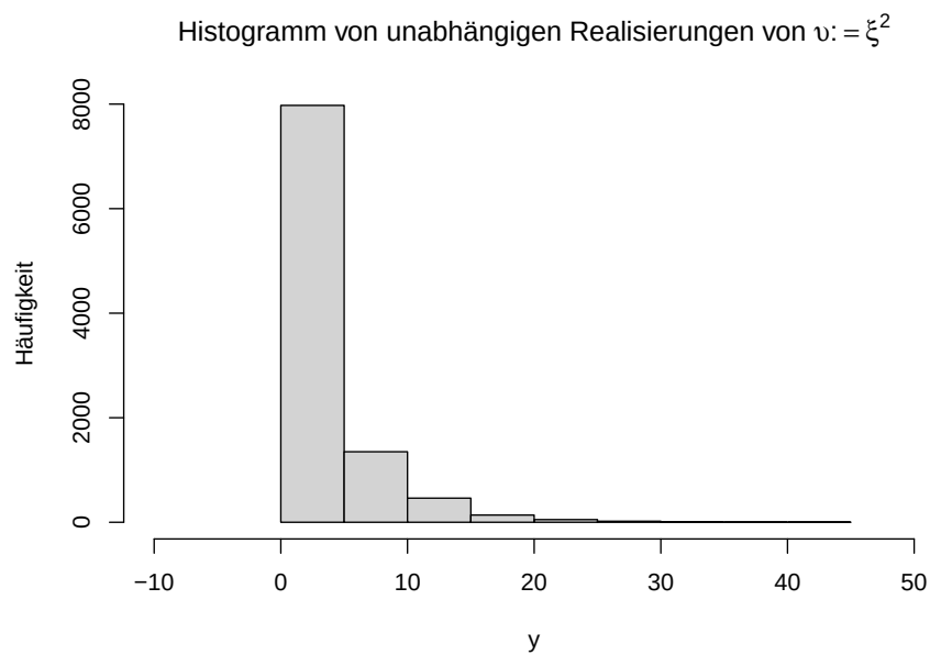
Abbildung 20.2. Histogramm von 10.000 quadrierten Realisierungen unabhängig und identisch normalverteilter Zufallsvariablen.
