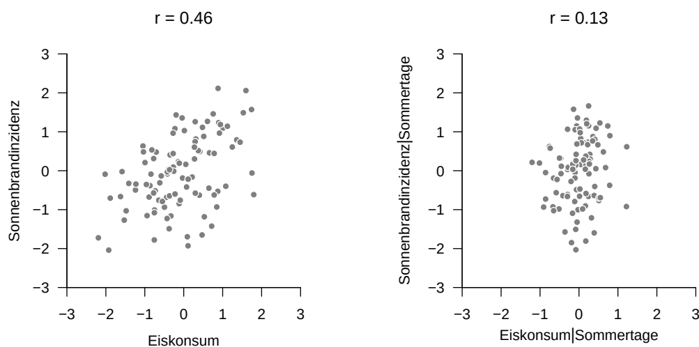
Abbildung 35.3. Evaluation der partiellen Korrelation im Beispielszenario.
