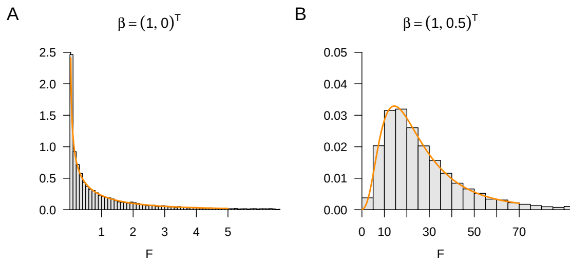
Abbildung 31.2. Exemplarische F-Statistik Verteilungen unter reduziertem und vollständigem wahren, aber unbekannten, datenerzeugenden Modell bei einfacher linearer Regression.
