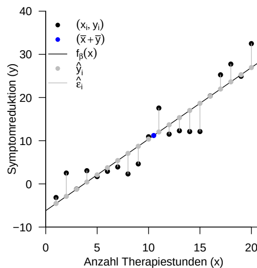
Abbildung 27.3. Ausgleichsgerade, erklärte Werte und Residuen für den Beispieldatensatz..
