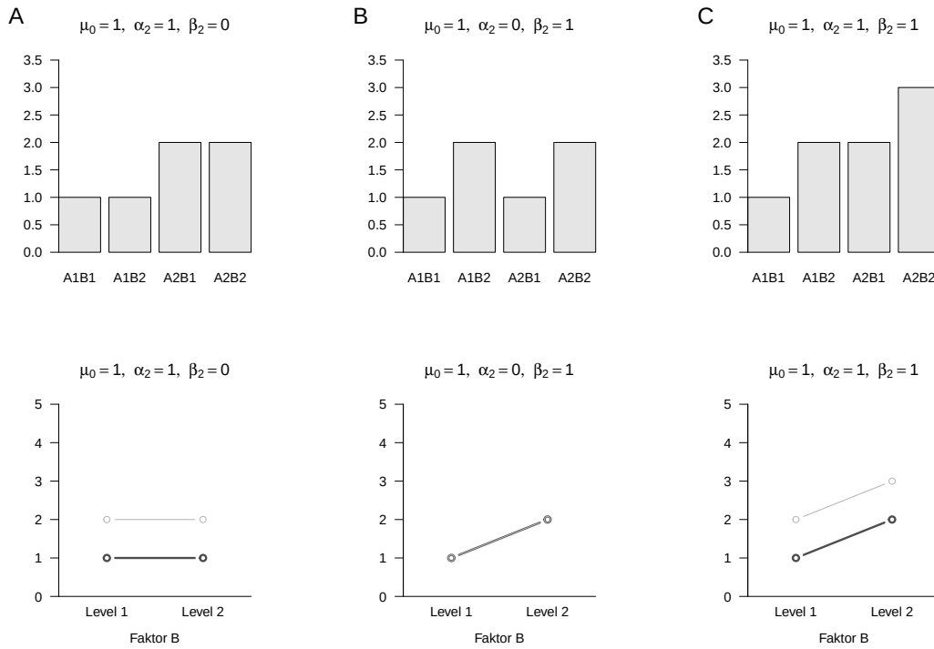
Abbildung 34.4. Gruppenerwartungswerte der Beispielparameterszenarien in Balken- und Liniendiagrammform im Modell der additiven ZVA.
