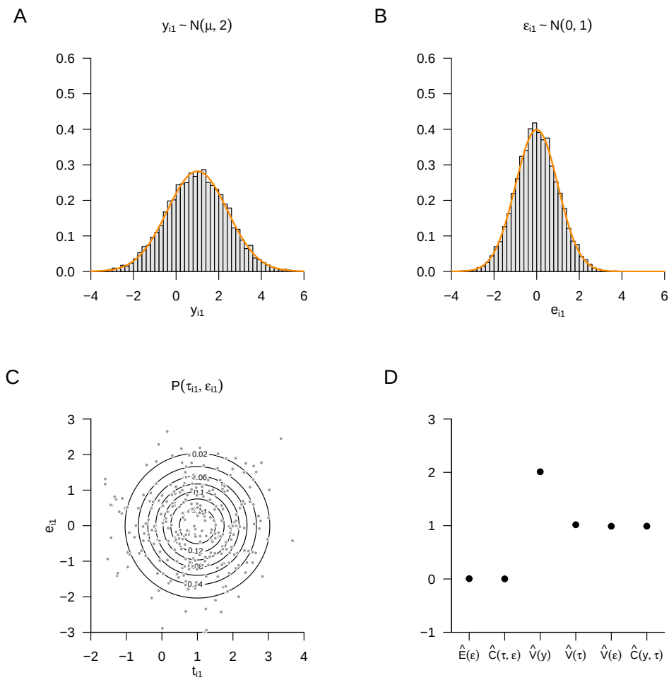
Abbildung 42.1. Normalverteilungsbeispiel bezüglich einer Testmessung.
