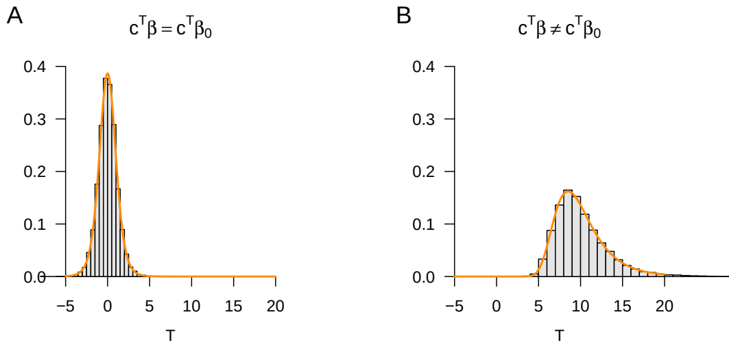
Abbildung 30.2. Verteilungen der T-Statistik bei einfacher linearer Regression.
