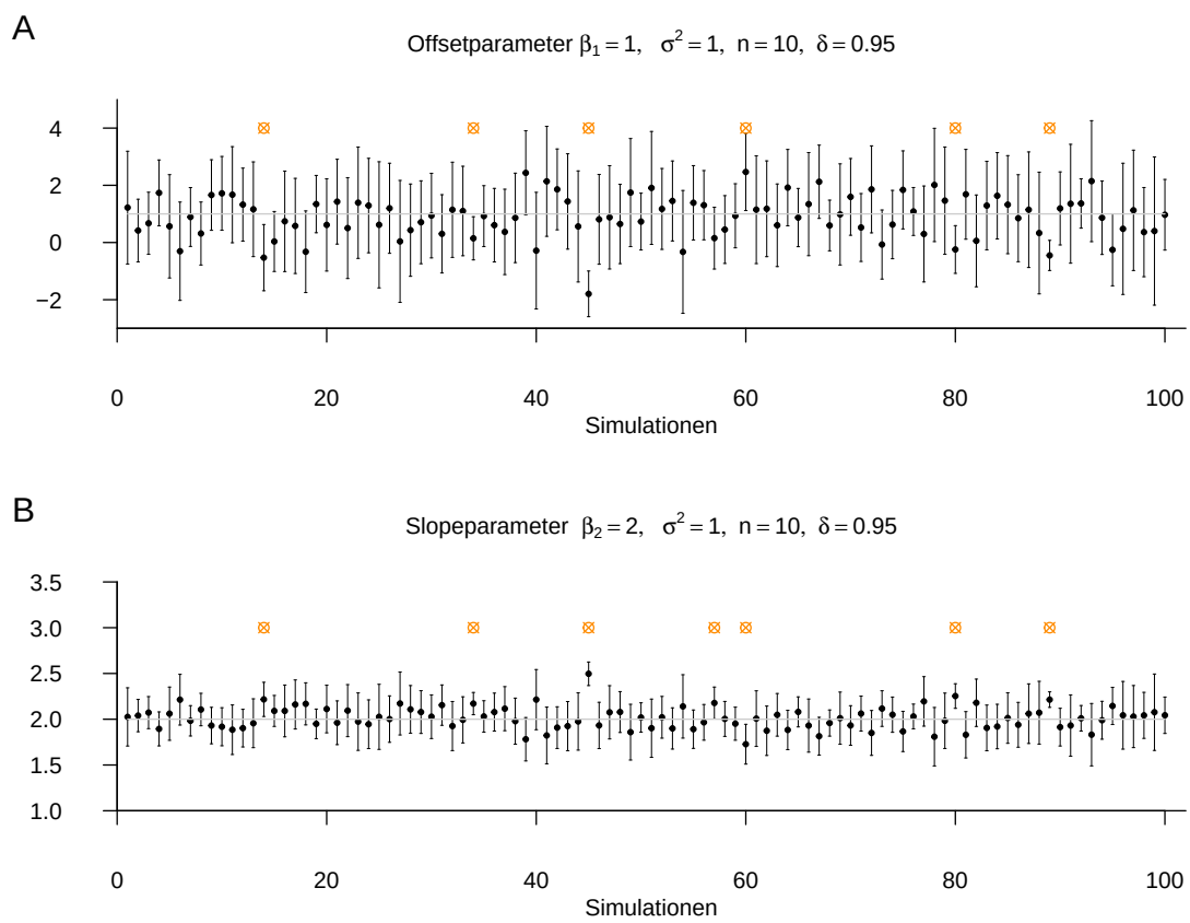
Abbildung 30.3. Konfidenzintervalle für Betaparameterkomponenten bei einfacher linearer Regression.
