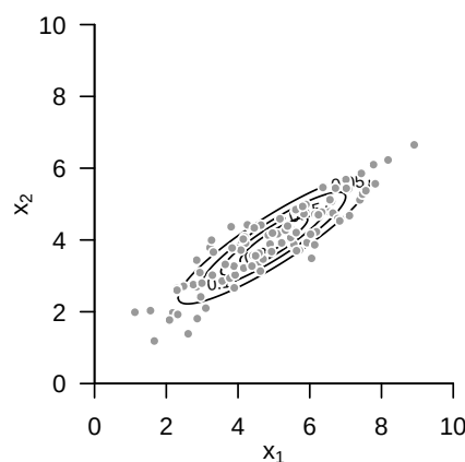
Abbildung 21.2. Konstruktion bivariater Normalverteilungen.
