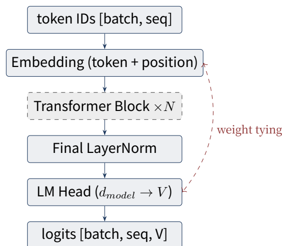
Figure 7.1: GPT 모델 구조. 임베딩 가중치와 LM Head 가중치를 공유(weight tying)하여 파라미터 절약.
