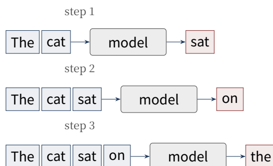
Figure 8.1: 자기회귀 생성 과정. 매 스텝마다 이전 토큰들을 모델에 넣고 다음 토큰을 예측.
