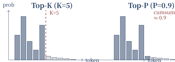
Figure 8.3: Top-K vs Top-P. Top-K는 고정 개수를, Top-P는 누적 확률이 P 가 될 때까지 선택.
