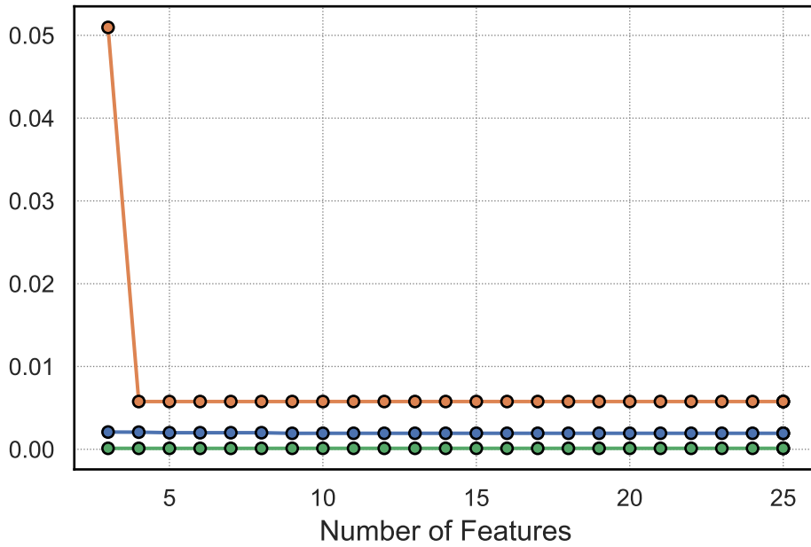
R^2
