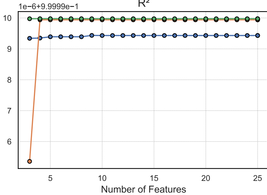
R^2
