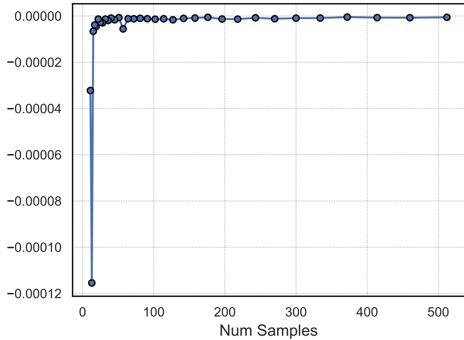
R^2
