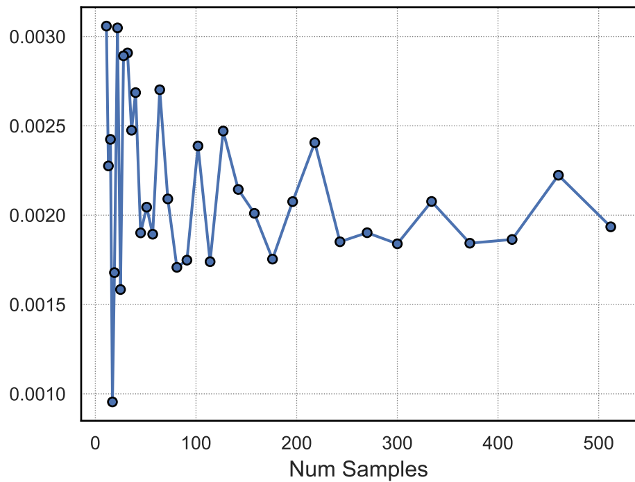
R^2
