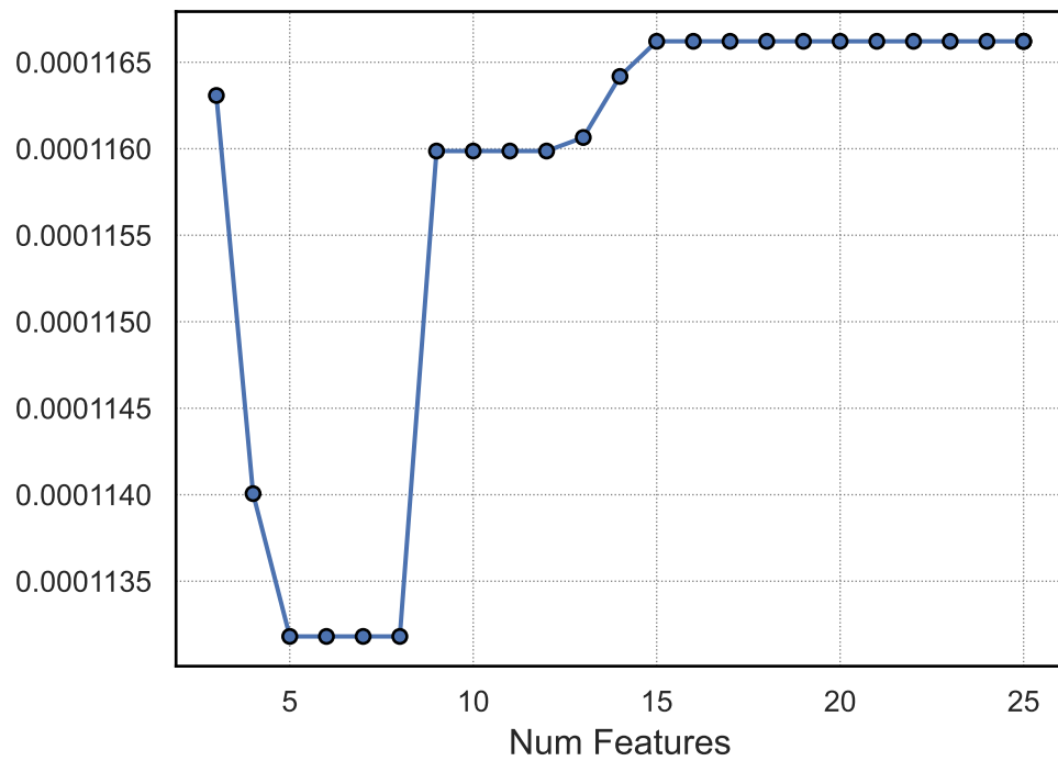
R^2
