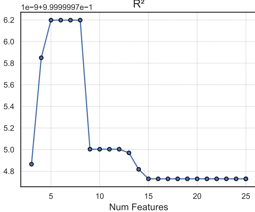
R^2
