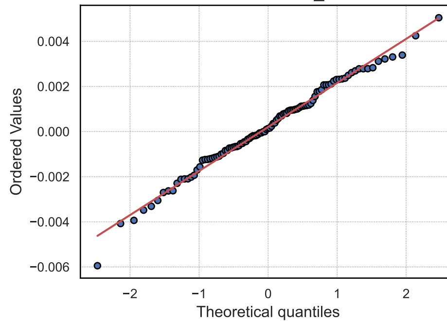
QQ-Plot: elastic_net
