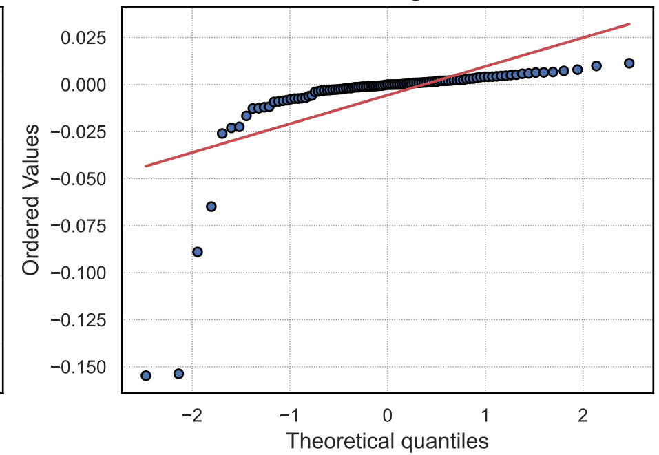
QQ-Plot: xgboost
