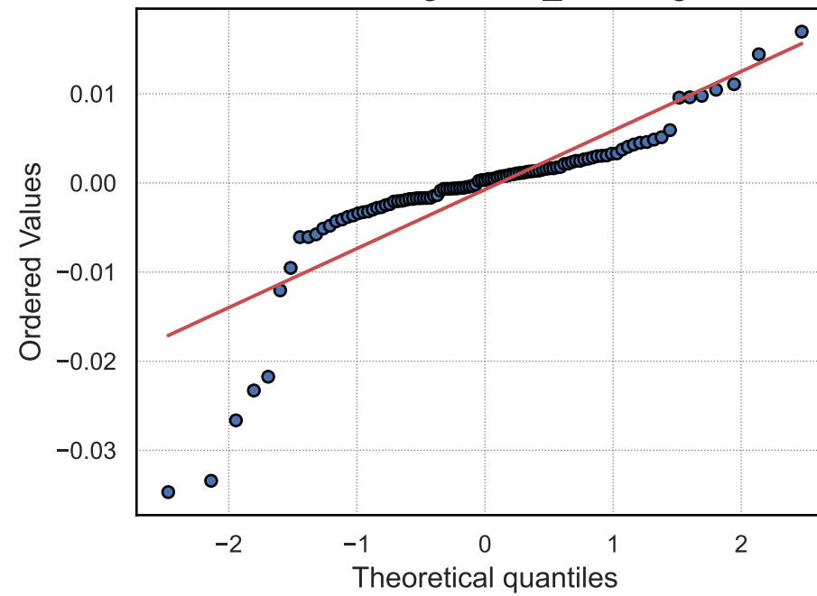
QQ-Plot: elastic_net
