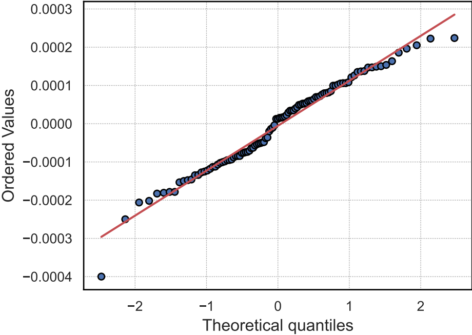
QQ-Plot: elastic_net
