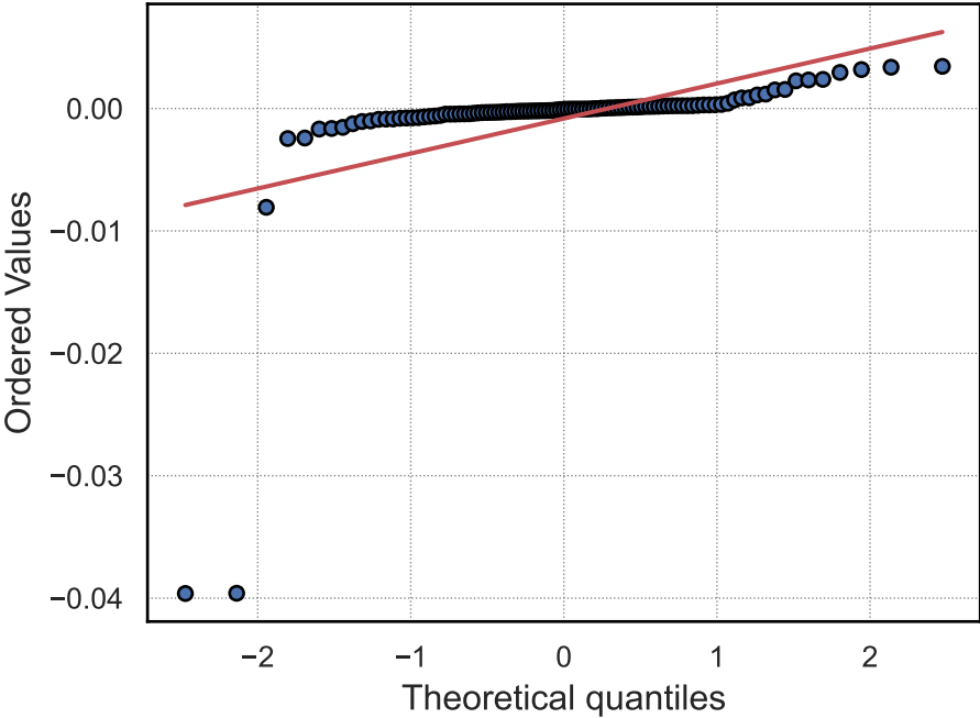
QQ-Plot: elastic_net
