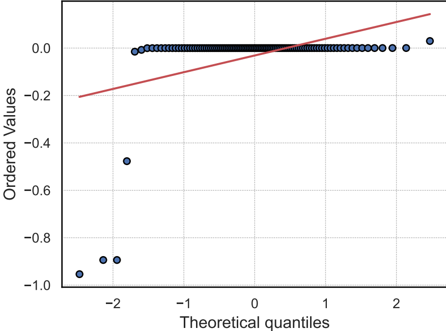
QQ-Plot: xgboost
