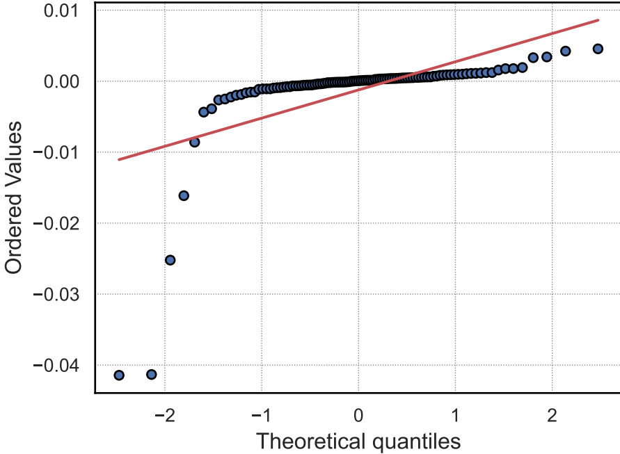
QQ-Plot: xgboost
