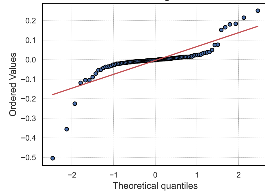
QQ-Plot: xgboost
