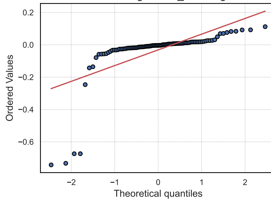
QQ-Plot: elastic_net
