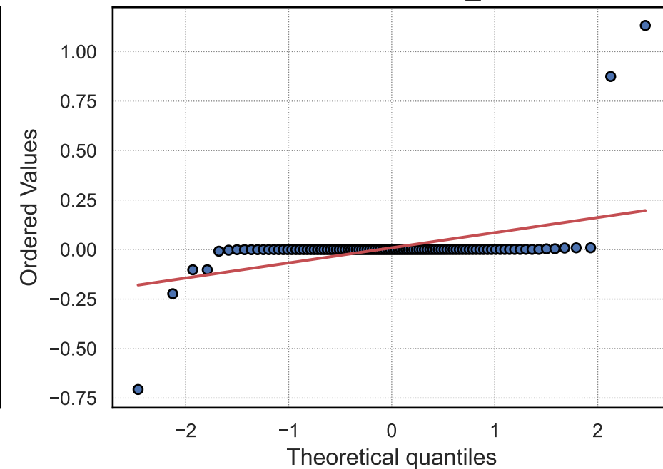
QQ-Plot: xgboost
