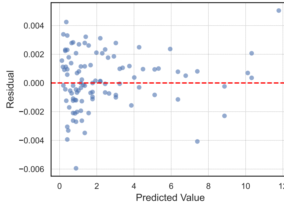
elastic_net
