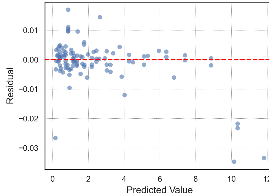
elastic_net
