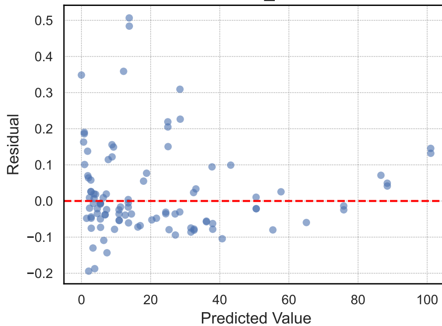
elastic_net
