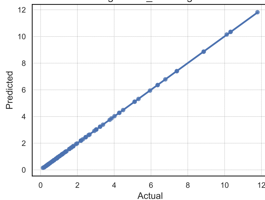
elastic_net
