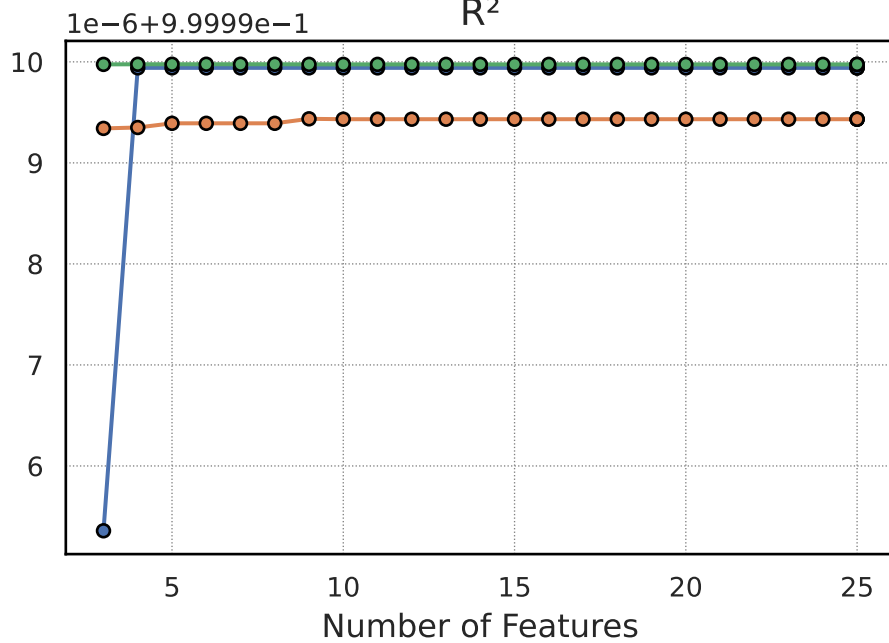
R^2
