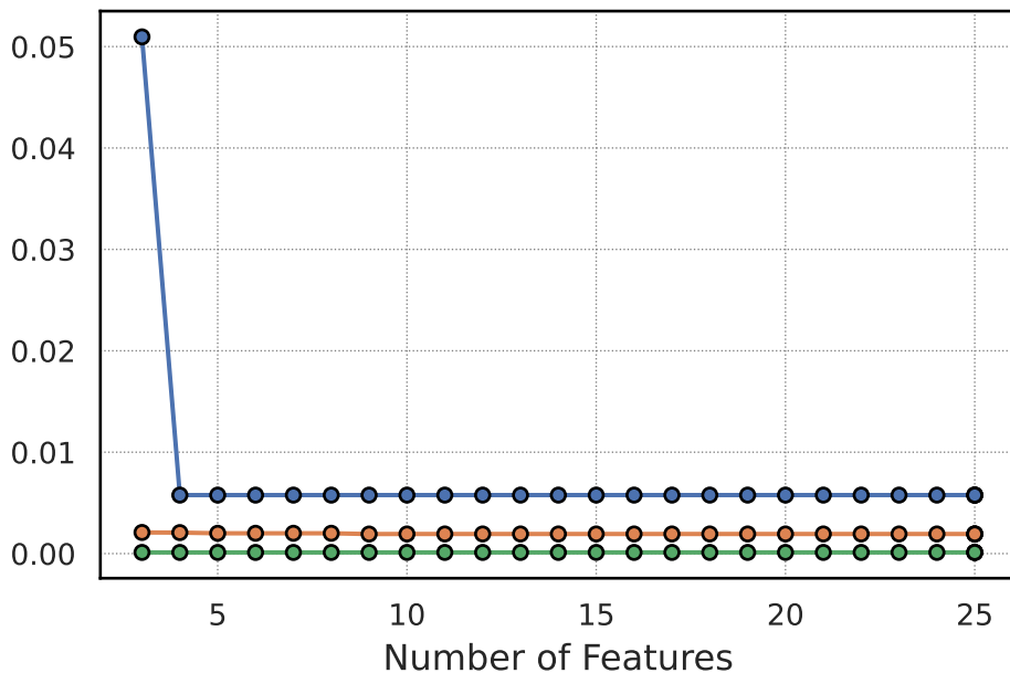
R^2
