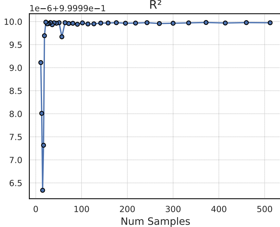
R^2
