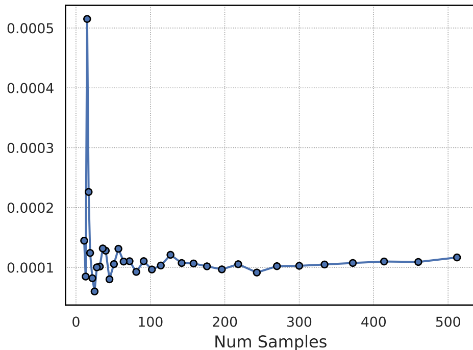
R^2
