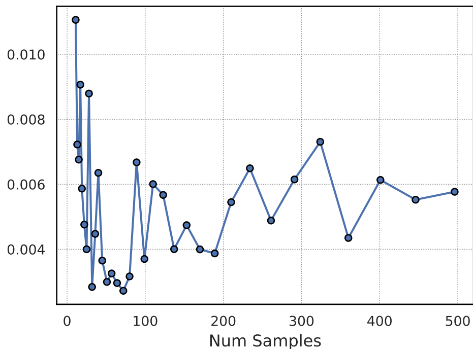
R^2
