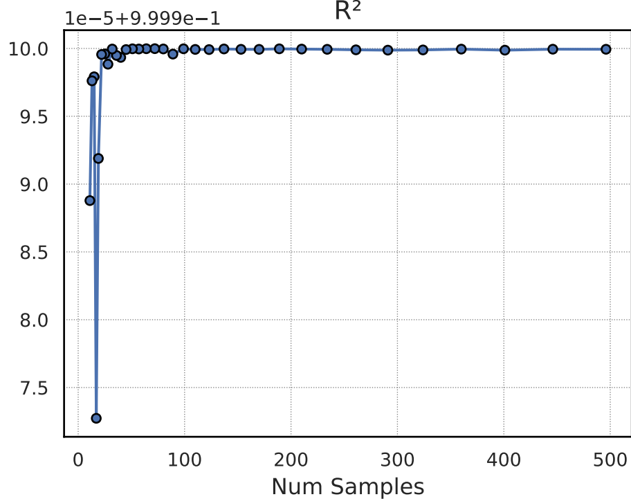
R^2
