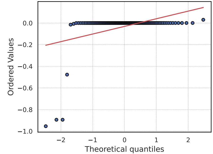
QQ-Plot: xgboost
