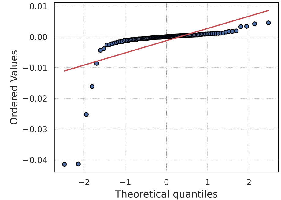
QQ-Plot: xgboost
