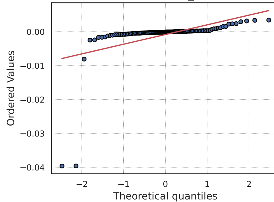
QQ-Plot: elastic_net
