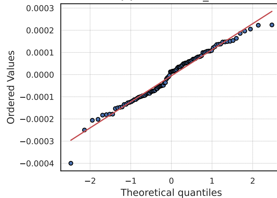
QQ-Plot: elastic_net
