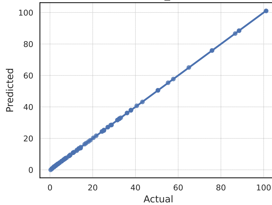
elastic_net
