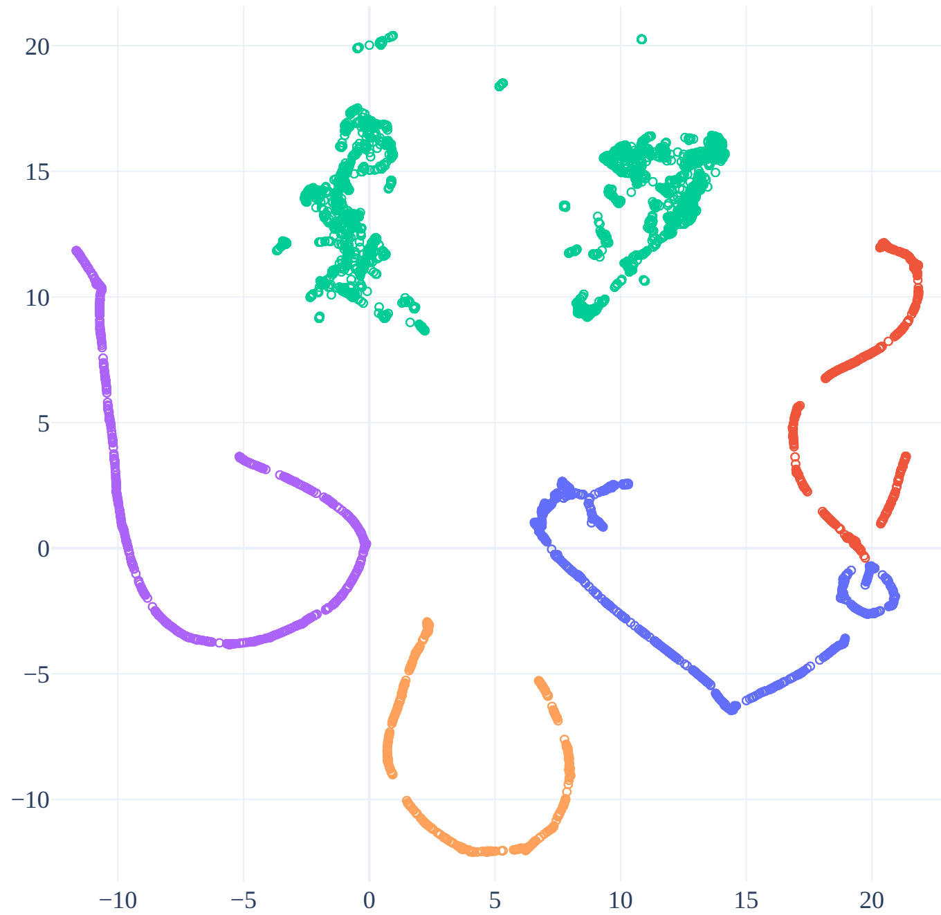
UMAP Scatter
