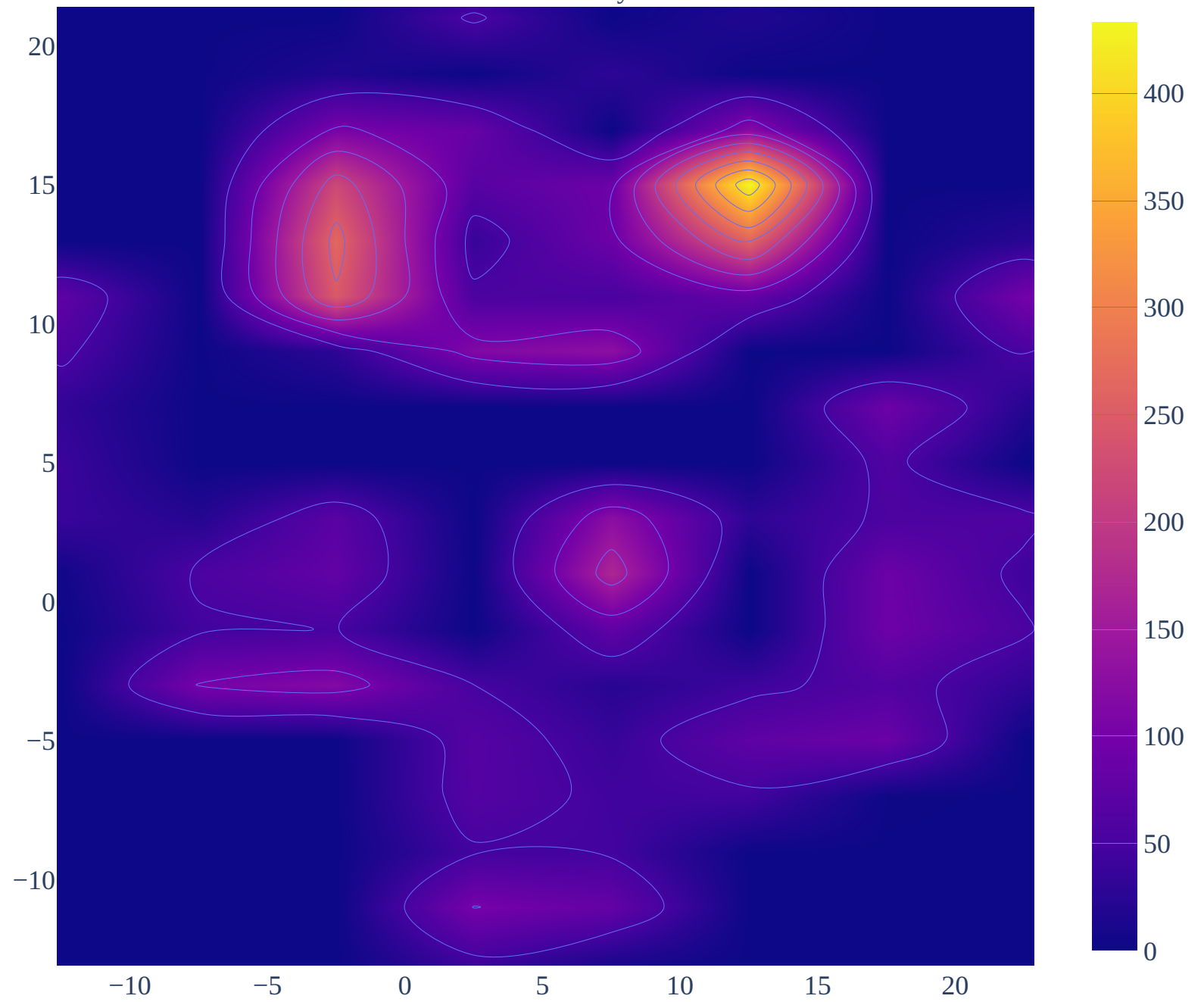
UMAP Density
