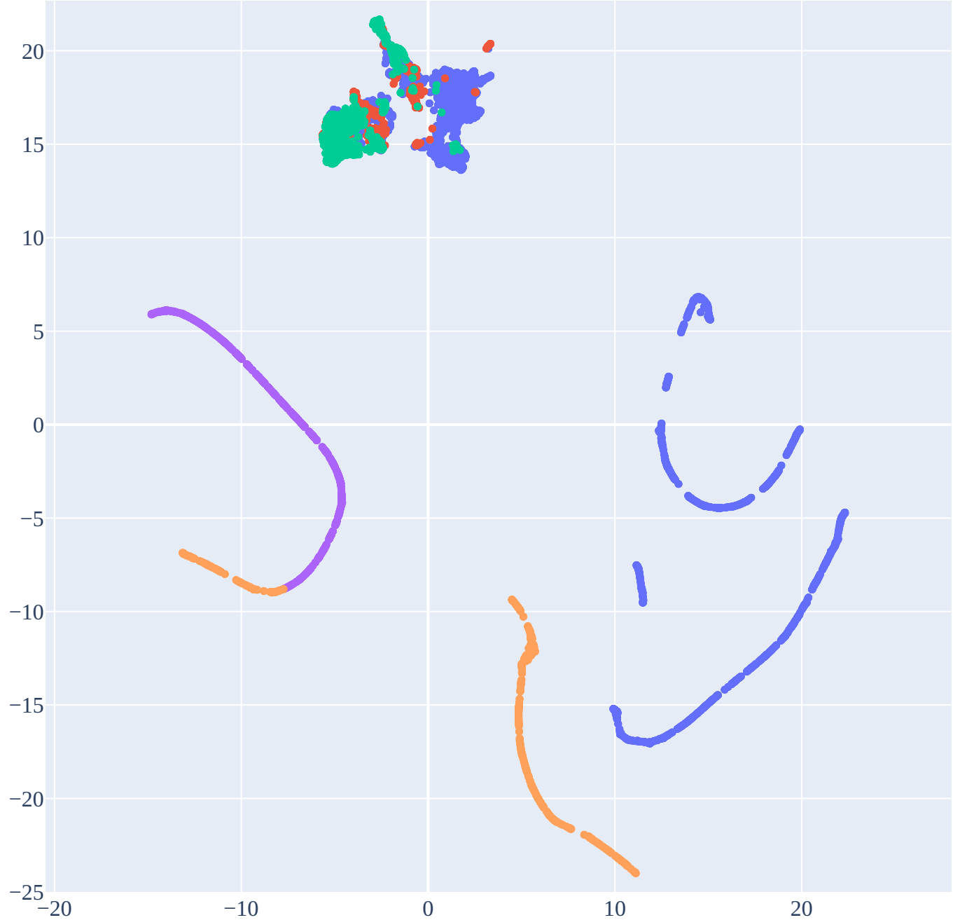
UMAP Scatter
