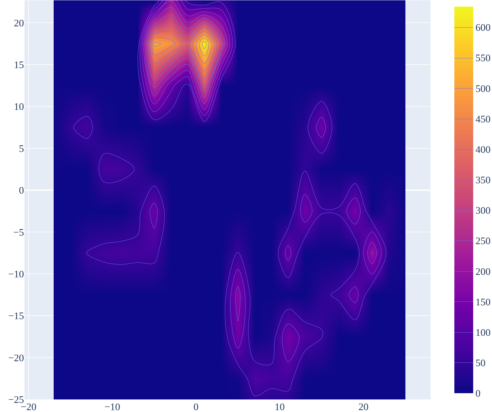
UMAP Density
