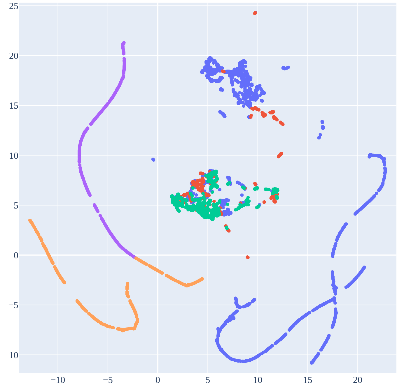
UMAP Scatter
