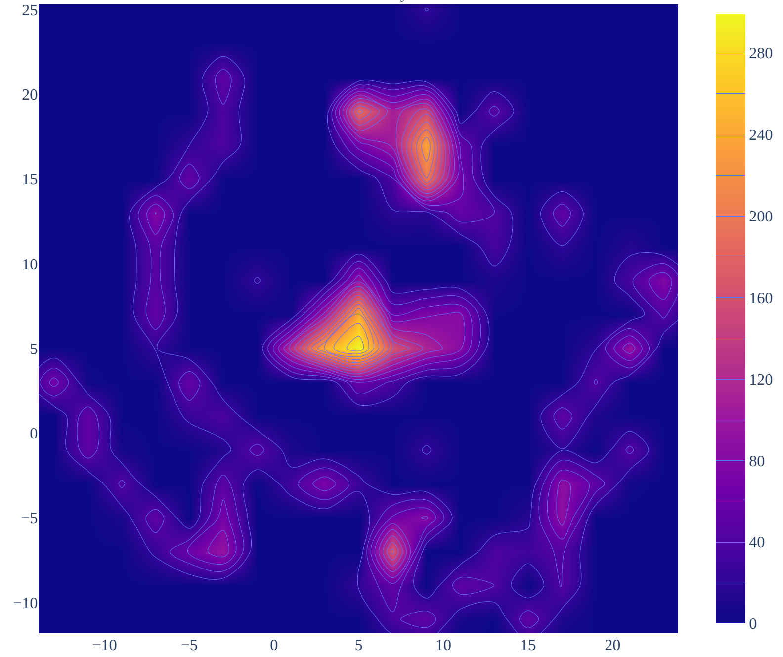
UMAP Density
