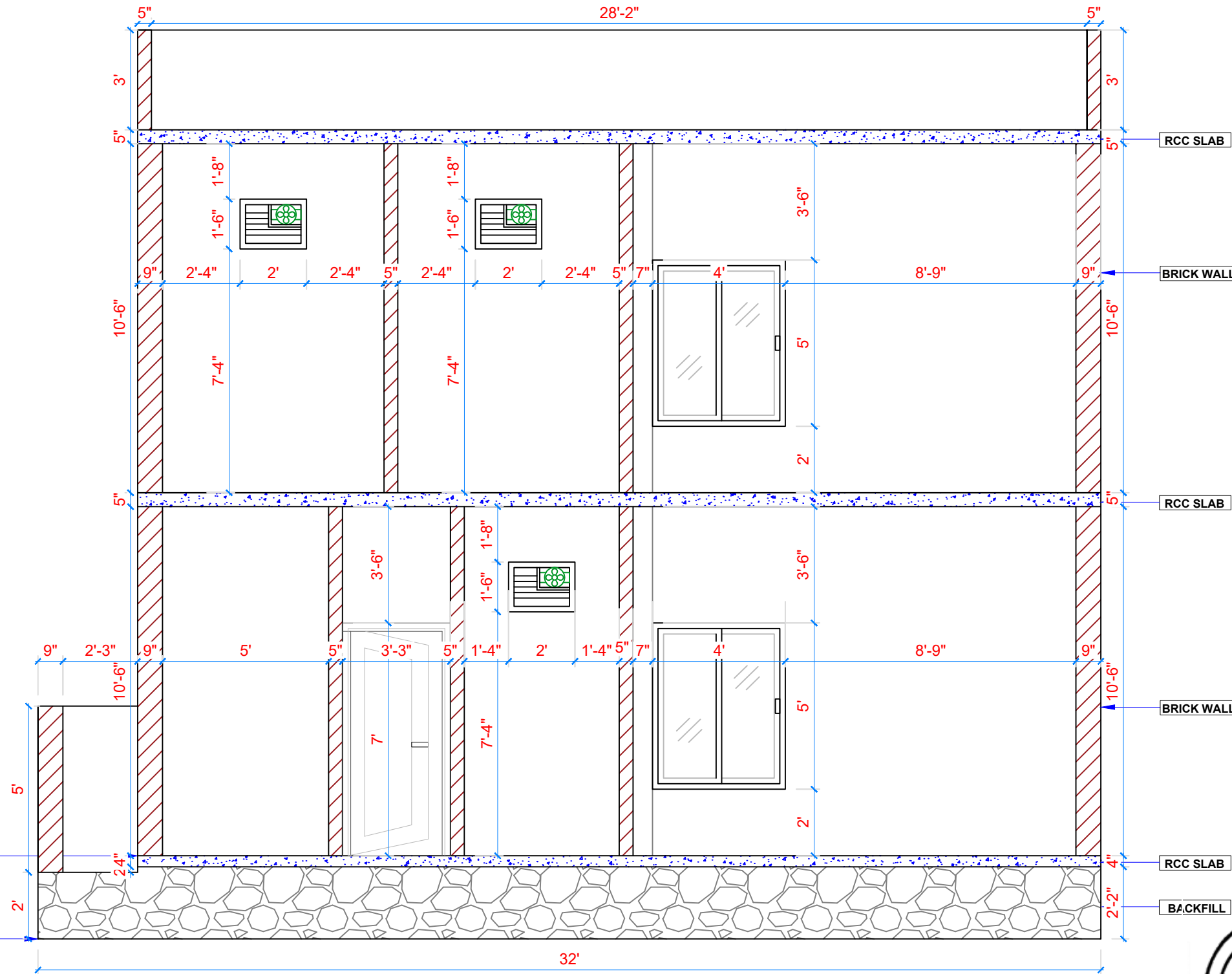
SECTION A-A'
