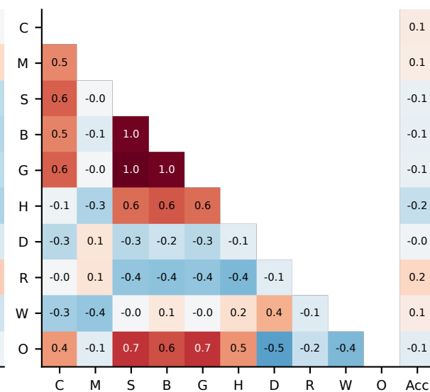
AIME25
