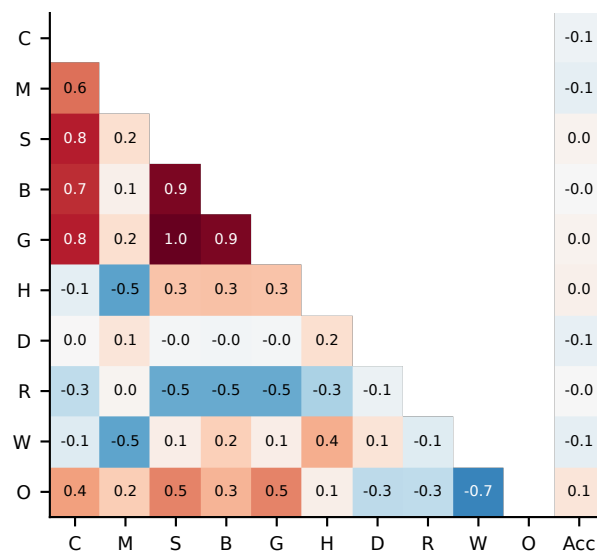
Minerva
