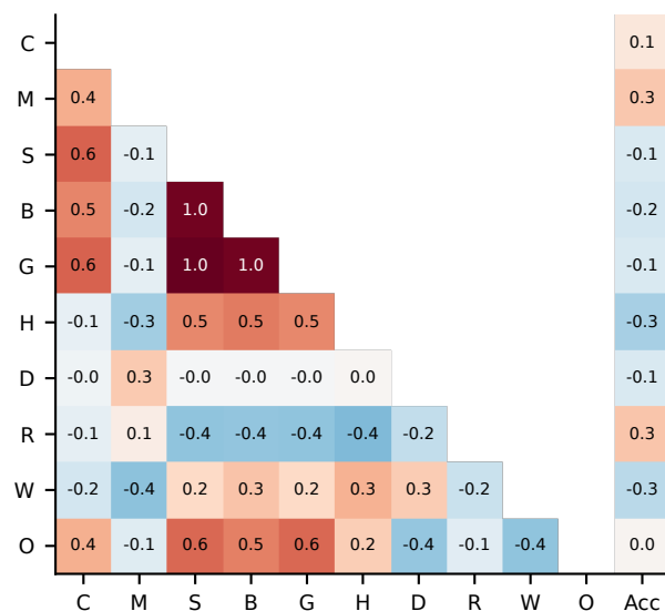
AIME24
