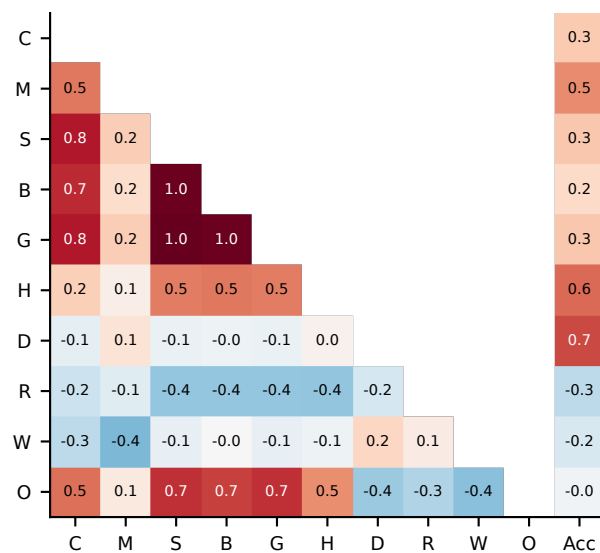
AMC23
