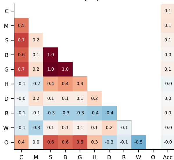
Olympiad
