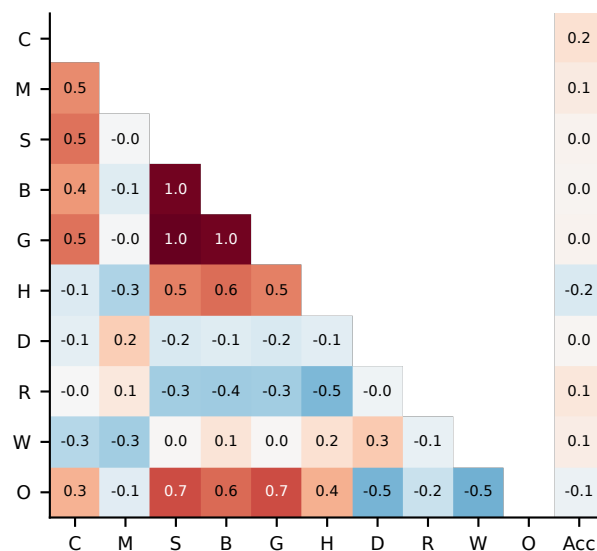
AIME25
