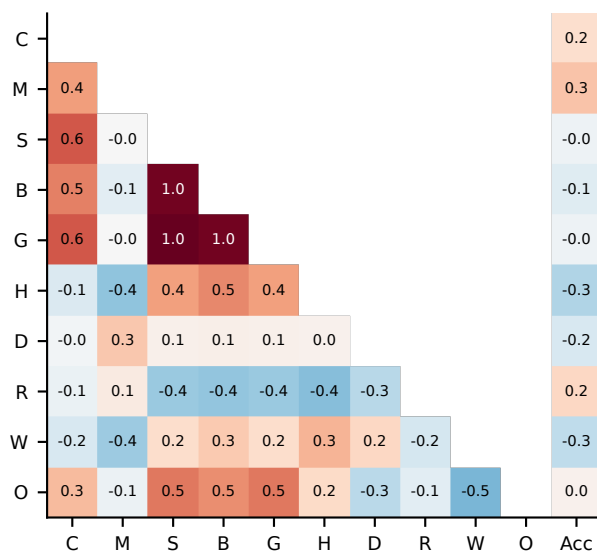
AIME24
