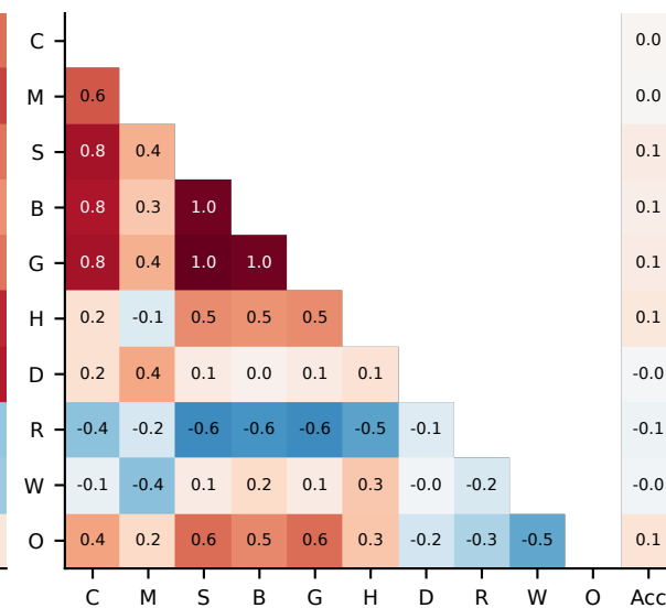
Minerva
