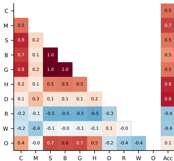
AMC23
