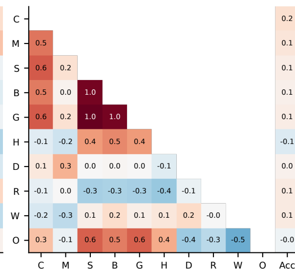
AIME25
