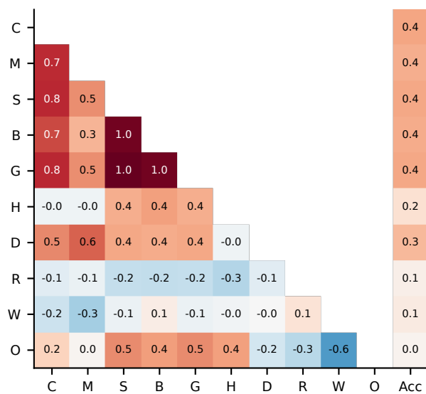
AIME25
