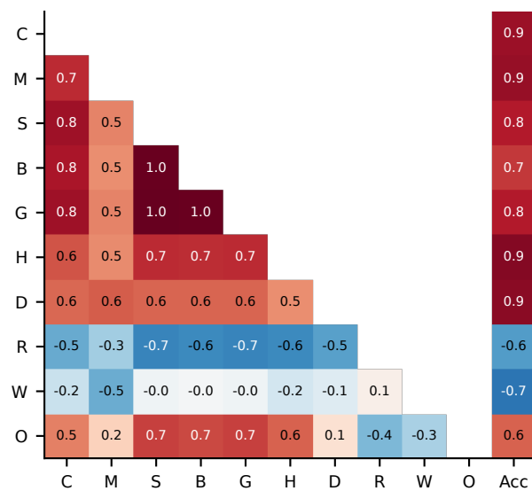
AMC23
