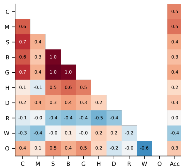
AIME24
