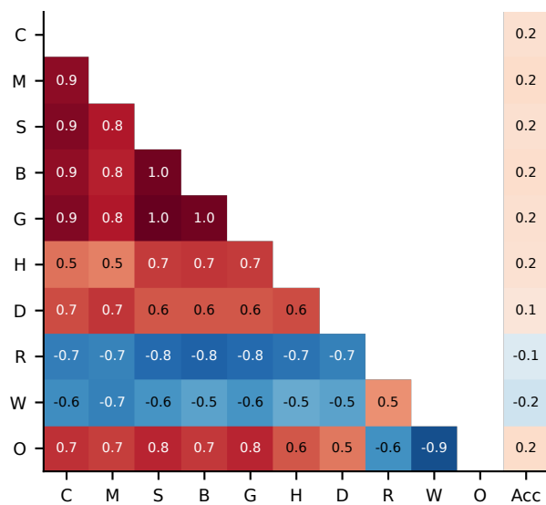
Minerva
