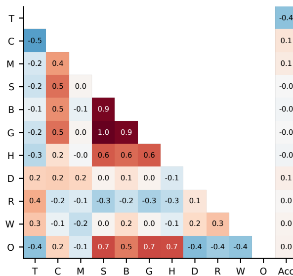
AIME25
