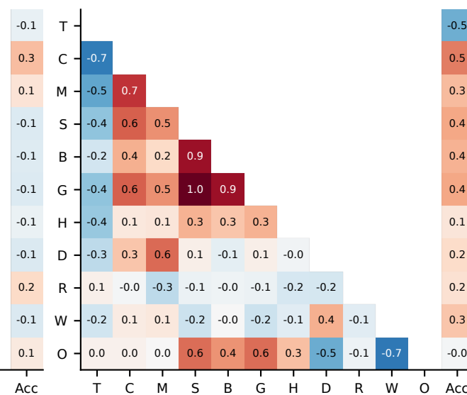
AIME25
