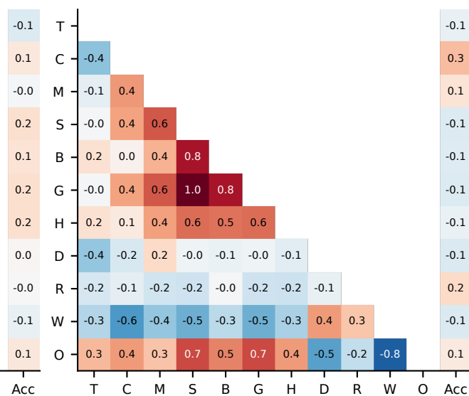
AIME24
