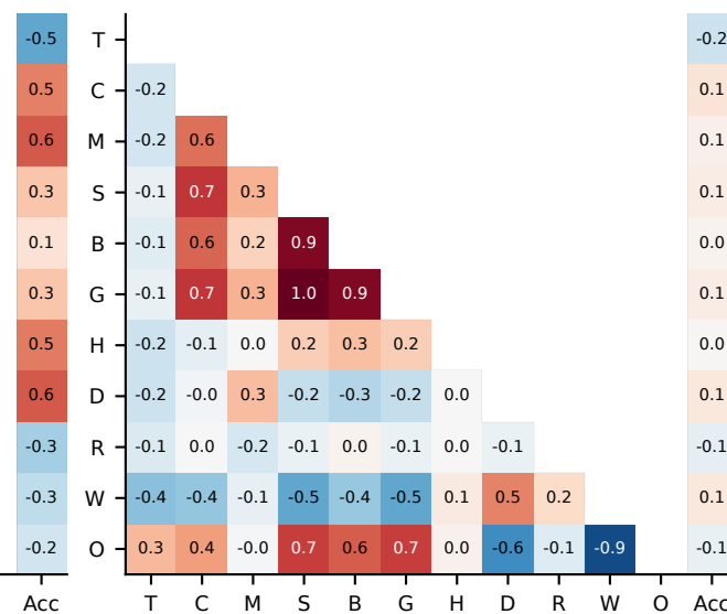
Minerva
