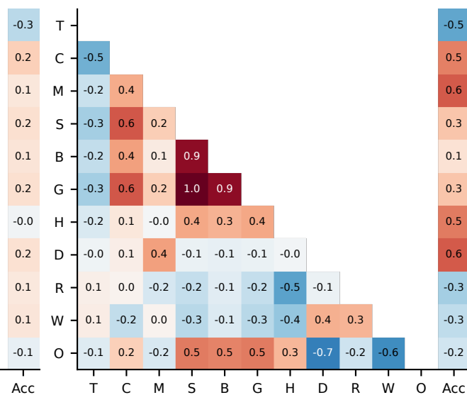
AMC23
