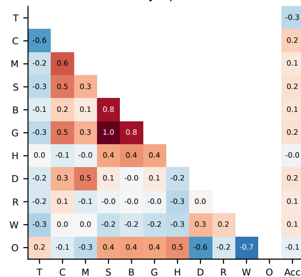
Olympiad
