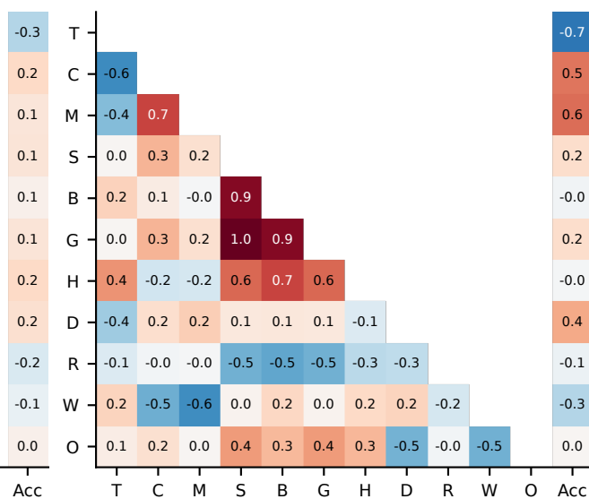
AIME24
