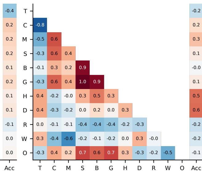
AMC23
