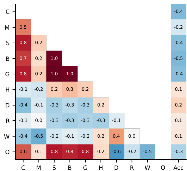
AMC23
