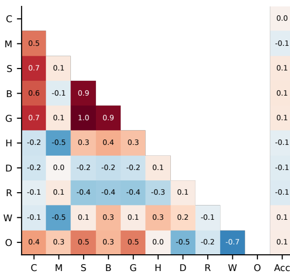
Minerva
