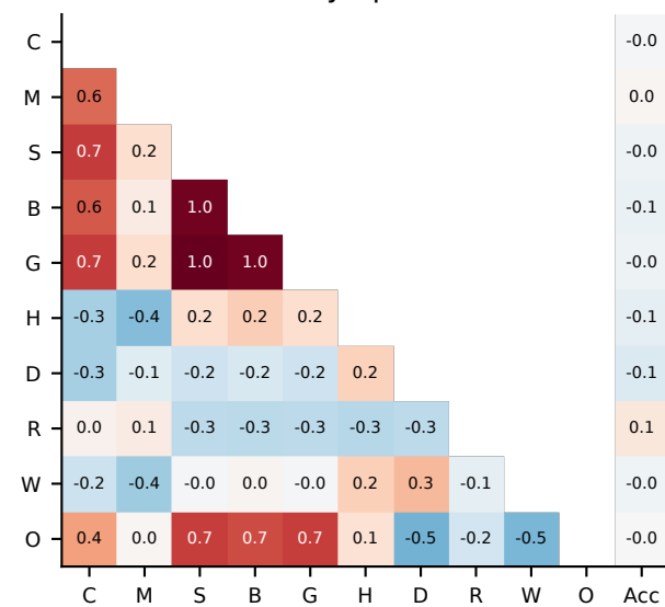
Olympiad
