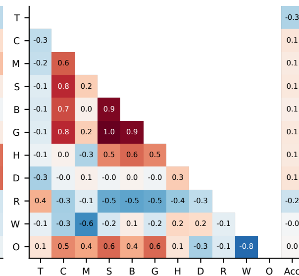
Minerva
