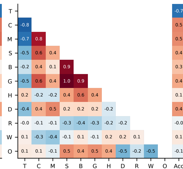
AIME25
