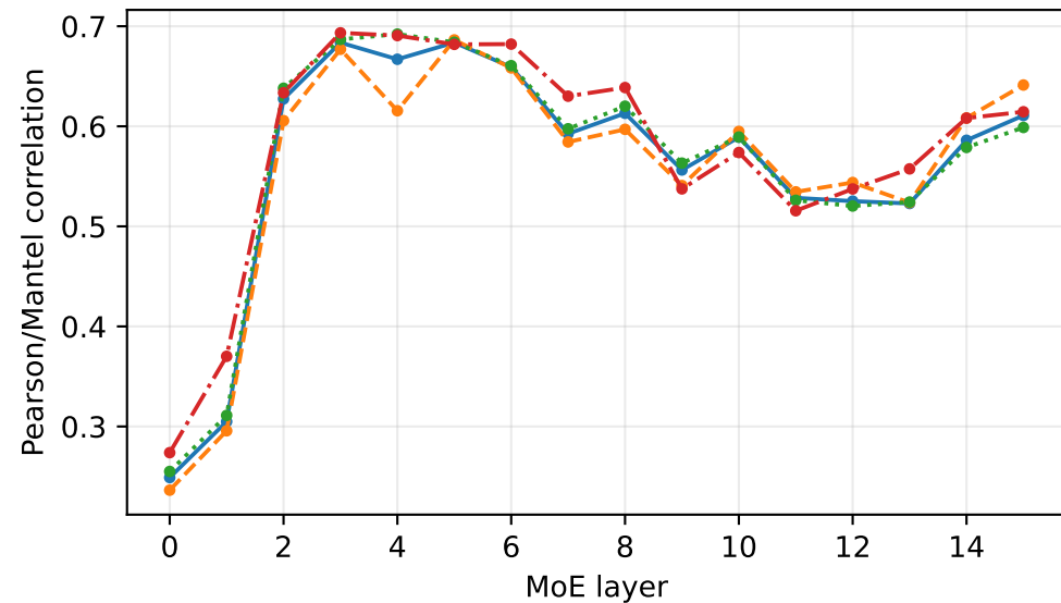
GSM8K
