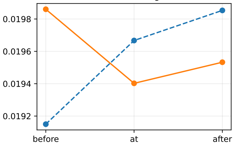
Router margin
