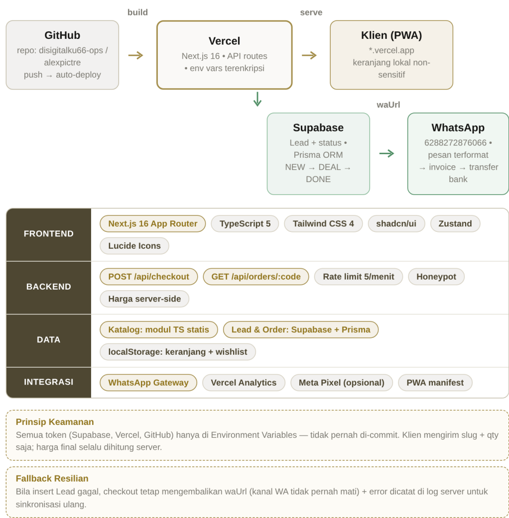
Gambar 6: Arsitektur deployment dan alur data — GitHub ke Vercel ke klien, dengan Supabase dan WhatsApp Gateway
