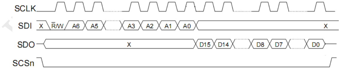
图 6 HSPI 寄存器读操作(大端模式)
