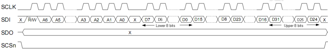
图 13 端口写操作(小端模式)
