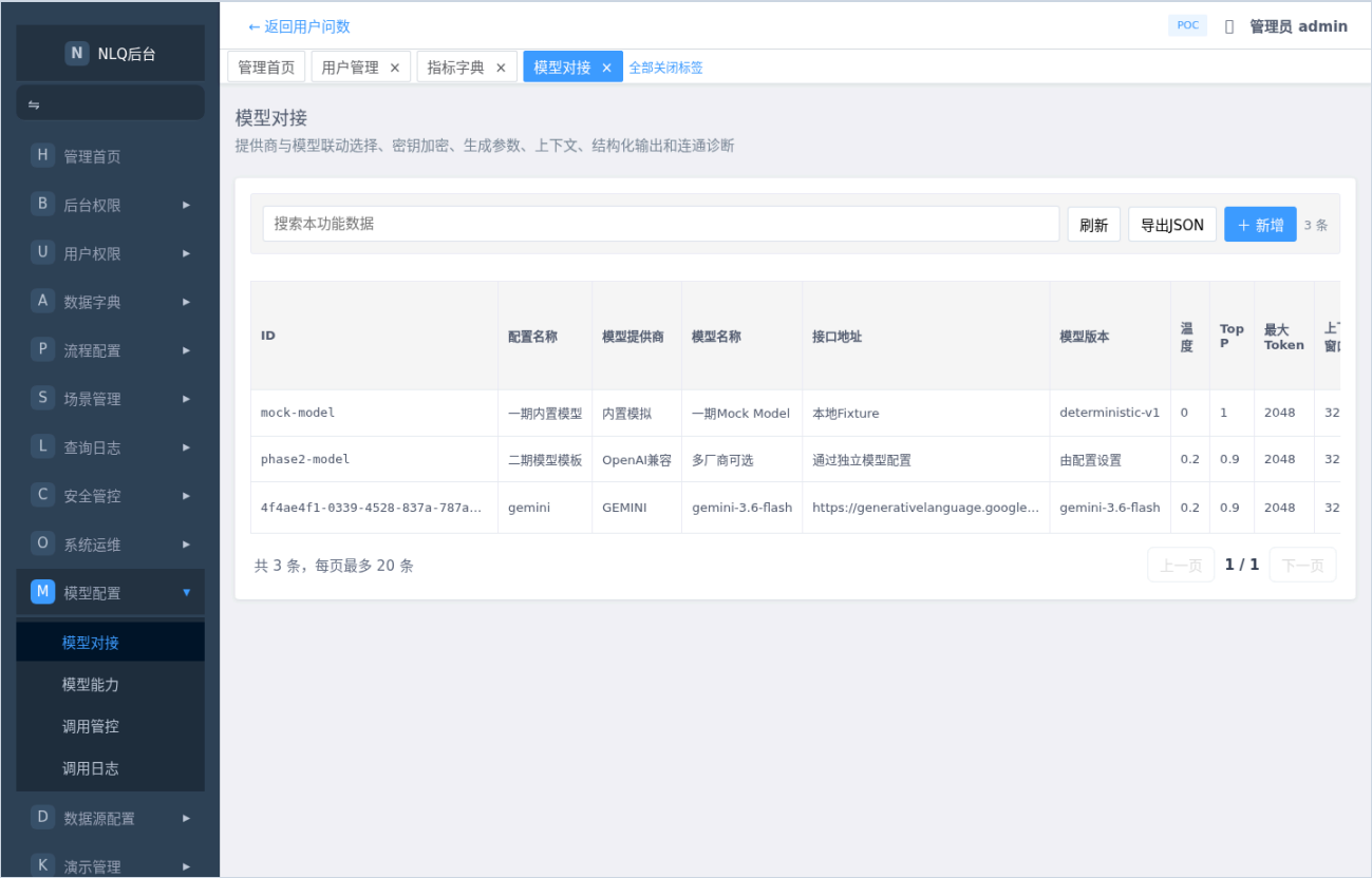
图4-4 模型配置
