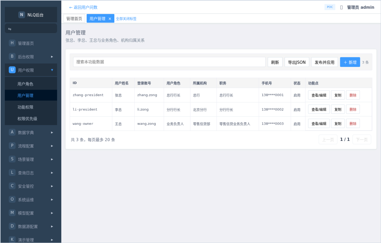
图4-2 用户管理
